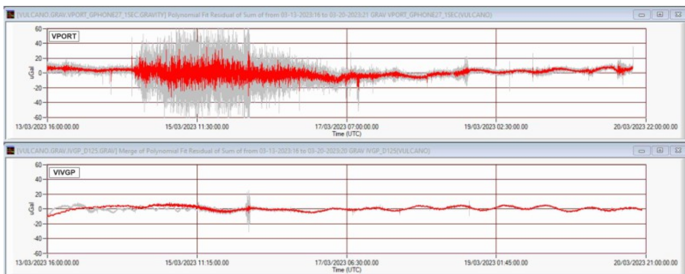
Fig. 13.1 Segnali gravimetrici registrati nelle stazioni VPORT (in alto) e VIVGP (in basso) dalle 16:00 UTC del 13 alle 20:00 UTC del 20 marzo 2023. In grigio segnali acquisiti al secondo; in rosso i segnali mediati al minuto. I dati sono corretti per gli effetti della marea terrestre e della deriva strumentale.
