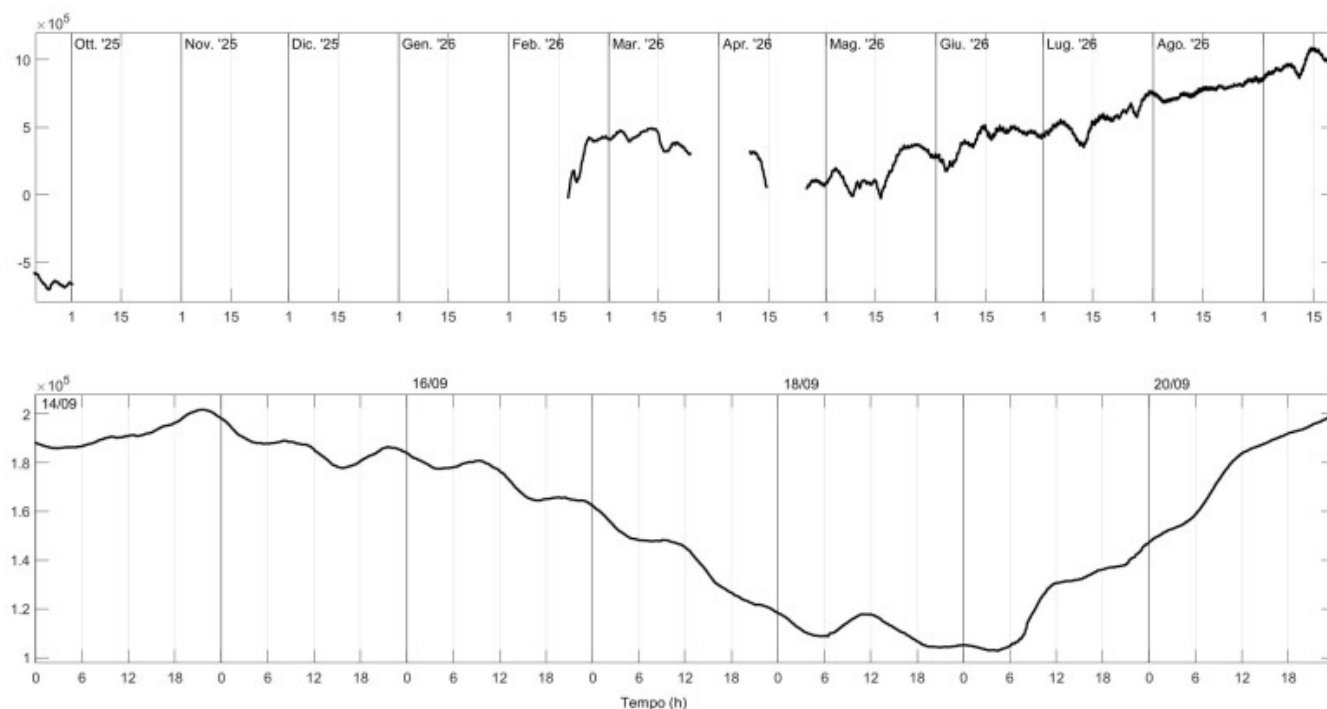
Fig. 4.3 Grafico relativo al dato dilatometrico registrato a SVO: in alto viene mostrato lo strain registrato nell'ultimo anno dal 21/09/2025; in basso quello registrato nell'ultima settimana.
