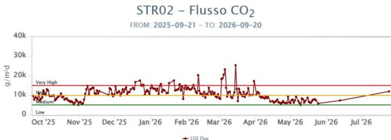
Fig. 6.2 Andamento del flusso CO 2 misurato sul Pizzo sopra la fossa, nell'ultimo anno
