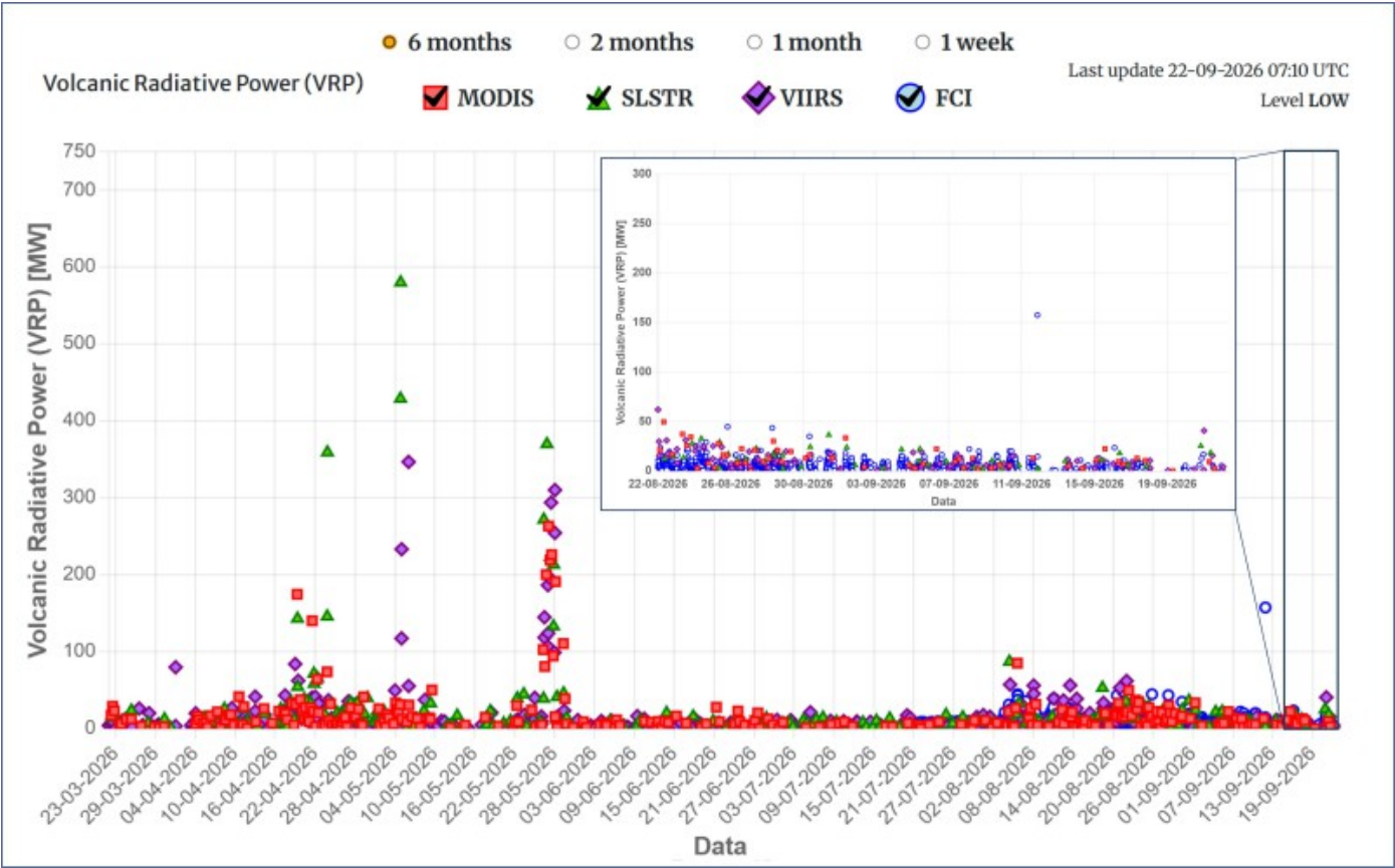
Fig. 7.1 Potere radiante calcolato da dati MODIS (quadrato rosso), SENTINEL-3 SLSTR (triangolo verde), VIIRS (triangolo viola e rombo giallo) e MTG-FCI (triangolo blu) dal 22 marzo 2026 al 22 settembre 2026. (riquadro) Potere radiante calcolato nell'ultima settimana https://www.ct.ingv.it/technolab/volchazard .
