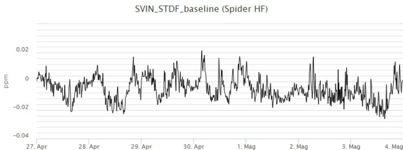
Fig. 5.1 Serie temporale della variazione di distanza tra i caposaldi STDF e SVIN
