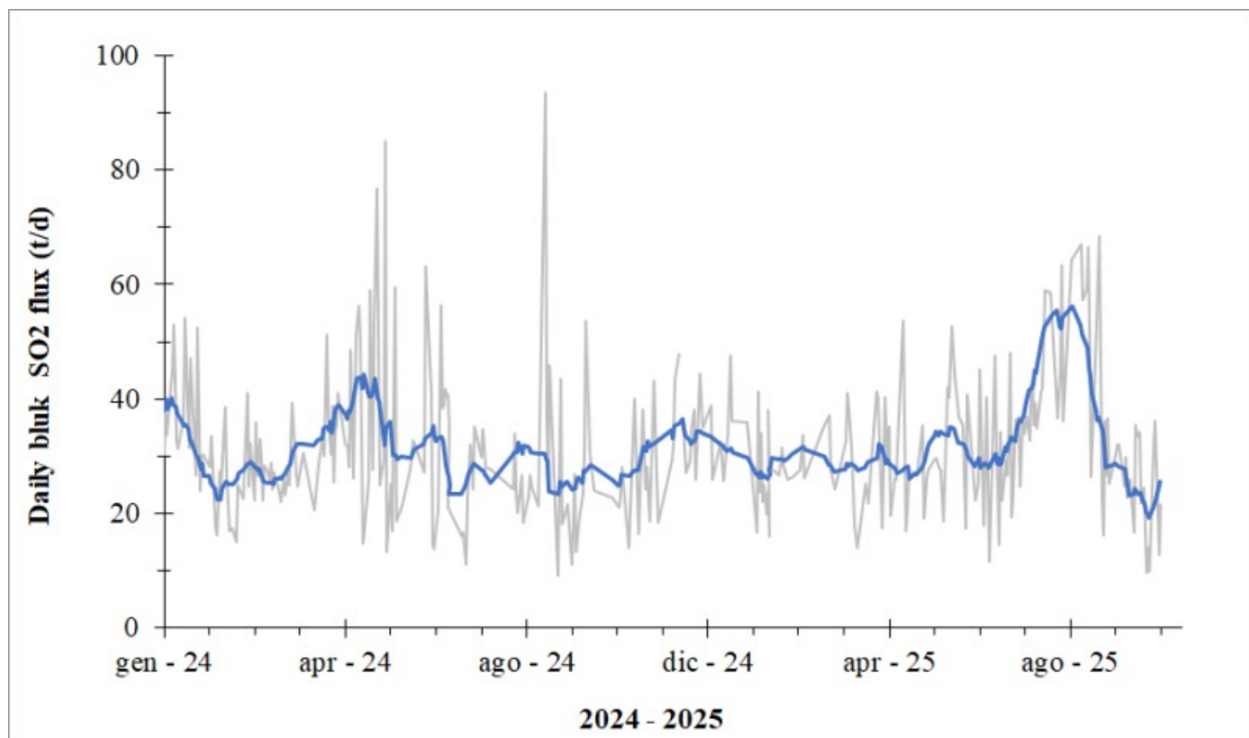
Fig. 5.1 Il flusso di SO 2 medio-giornaliero e medio-settimanale emesso dal campo fumarolico craterico di Vulcano nel periodo gennaio 2024 - 2 novembre 2025 (rispettivamente, linea grigia e blu)
