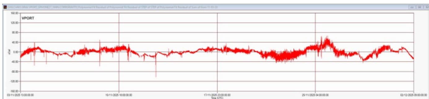
Fig. 13.1 Segnale gravimetrico registrato nella stazione VPORT dalle 13:00 UTC del 3 novembre alle 09:00 UTC del 02 dicembre 2025. Il segnale è mediato al minuto. I dati sono corretti per gli effetti della marea terrestre e della deriva strumentale.
