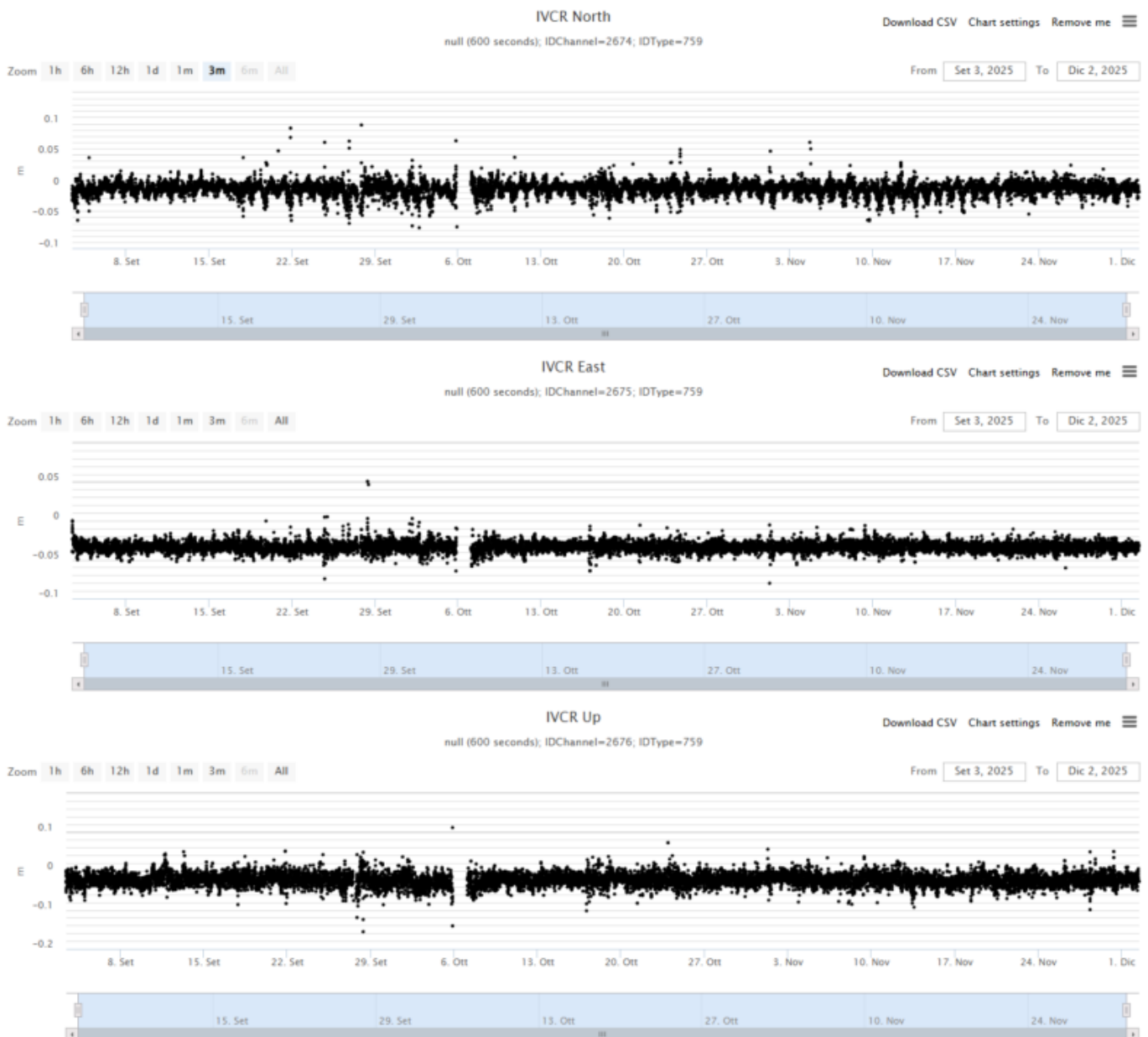
Fig. 11.1 Serie GNSS ad alta frequenza delle componenti orizzontali e verticale alla stazione di IVCR nel corso degli ultimi 3 mesi
