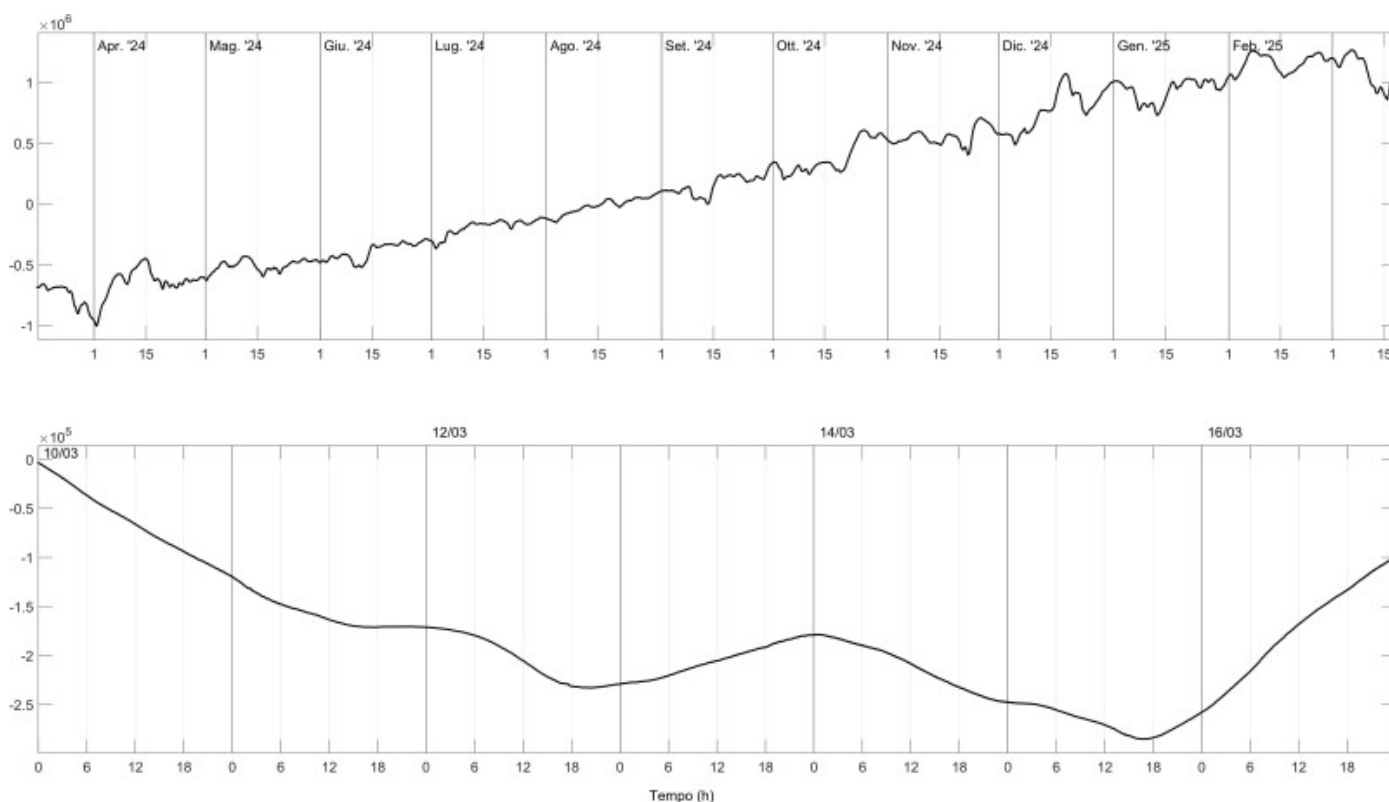
Fig. 4.3 Grafico relativo al dato dilatometrico registrato a SVO: in alto viene mostrato lo strain registrato nell'ultimo anno dal 17/03/2024; in basso quello registrato nell'ultima settimana.
