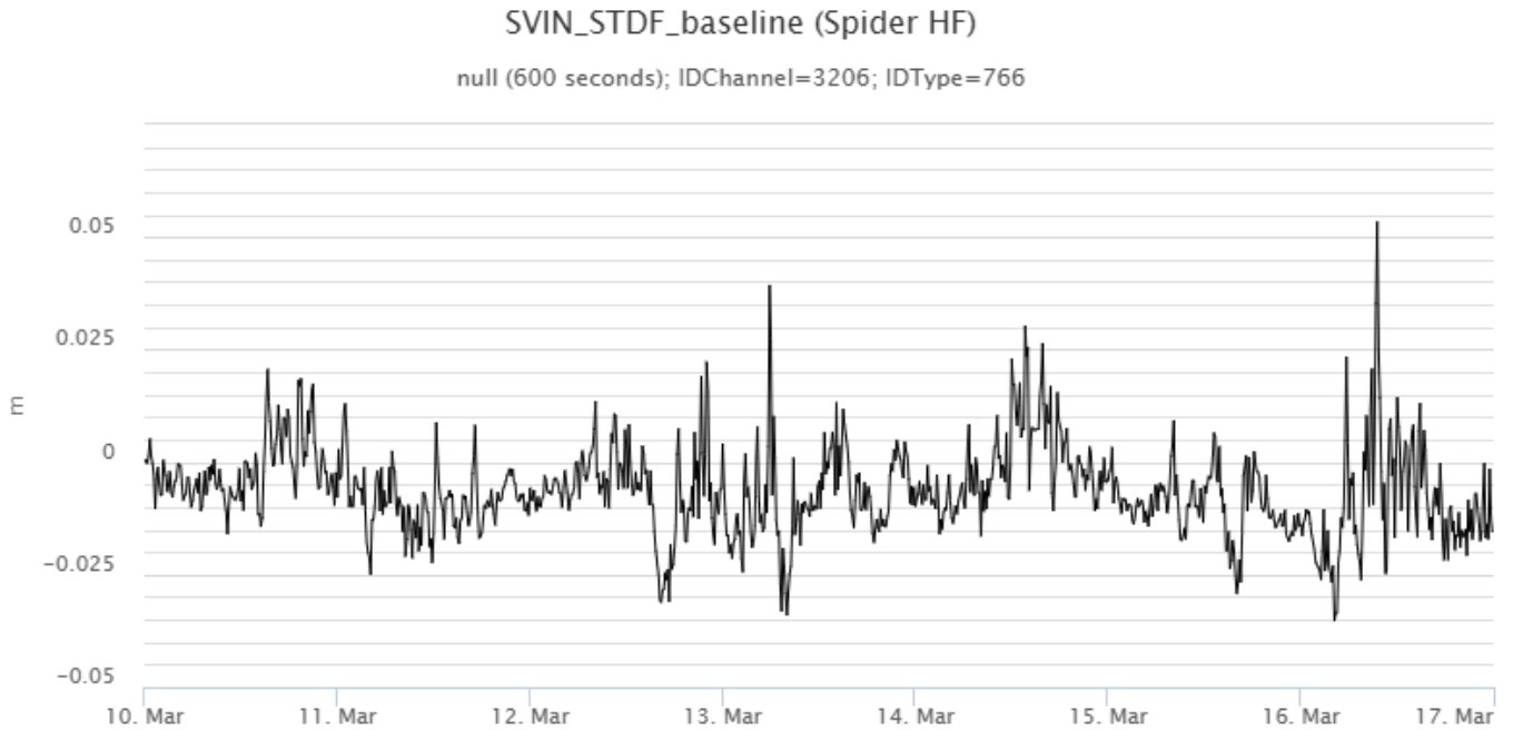
Fig. 5.1 Serie temporale della variazione di distanza tra le stazioni GNSS di San Vincenzo (SVIN) e di Timpone del Fuoco (STDF) nel corso dell'ultima settimana.
