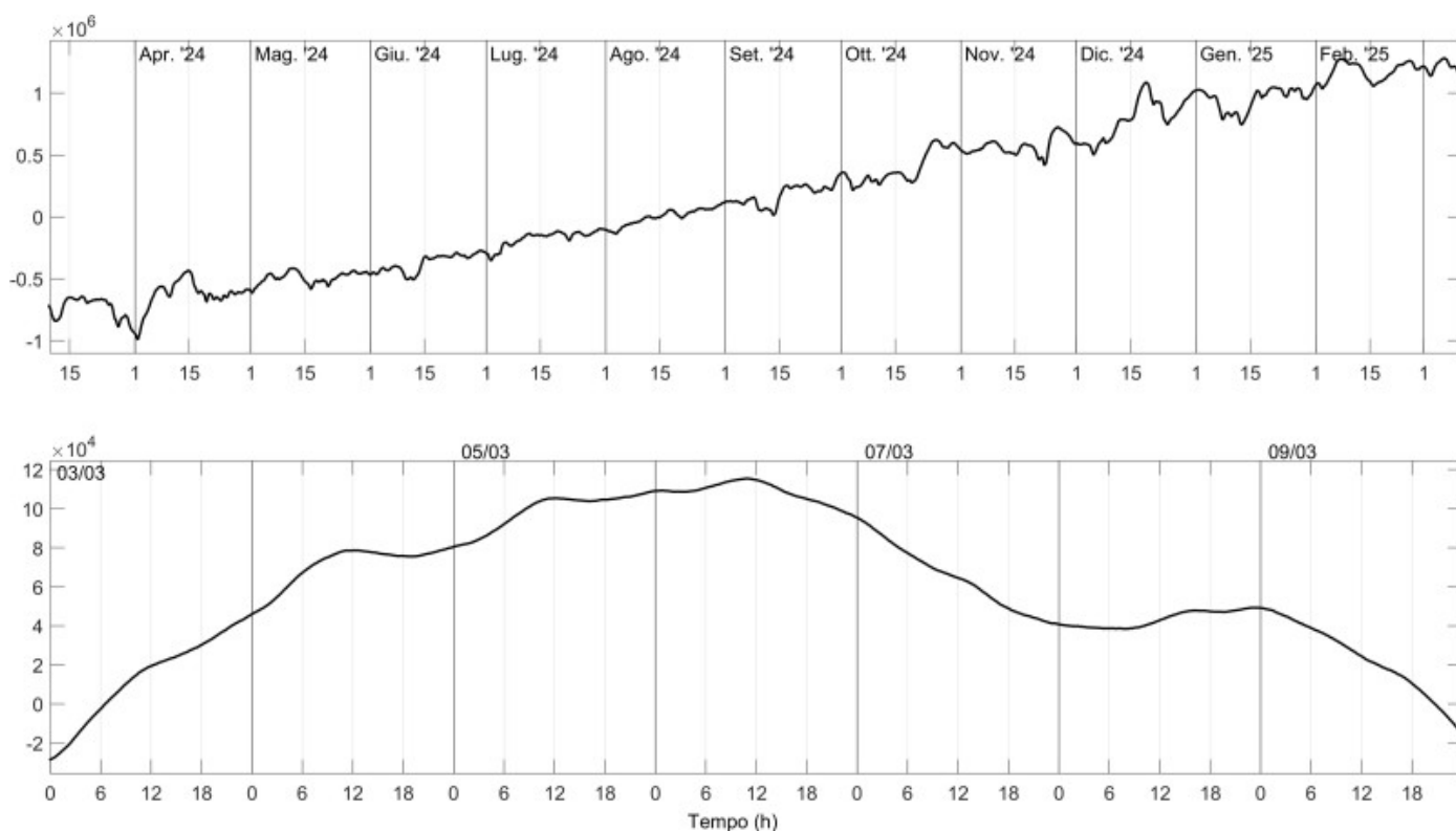
Fig. 4.3 Grafico relativo al dato dilatometrico registrato a SVO: in alto viene mostrato lo strain registrato nell'ultimo anno dal 10/03/2024; in basso quello registrato nell'ultima settimana.
