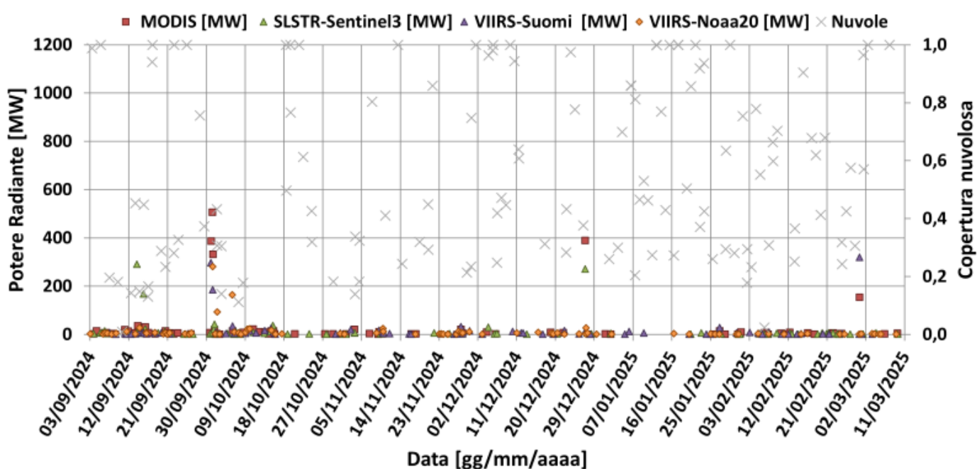
Fig. 7.1 Potere radiante calcolato da dati MODIS (quadrato rosso), SENTINEL-3 SLSTR (triangolo verde) e VIIRS (triangolo viola e rombo giallo) dal 3 settembre 2024 all'11 marzo 2025.
