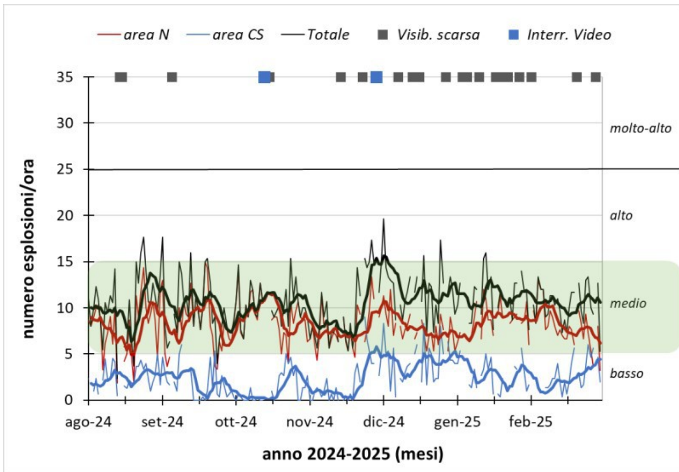
Fig. 3.2 Fig. 3.2 Frequenza media oraria giornaliera e settimanale per area craterica ed in totale dell'attività esplosiva dello Stromboli (rispettivamente linea sottile ed in grassetto). Al top del grafico è riportata la condizioni di osservazione del dato e a destra i livelli di attività; la barra verde indica il livello medio tipico dell'attività esplosiva dello Stromboli.
