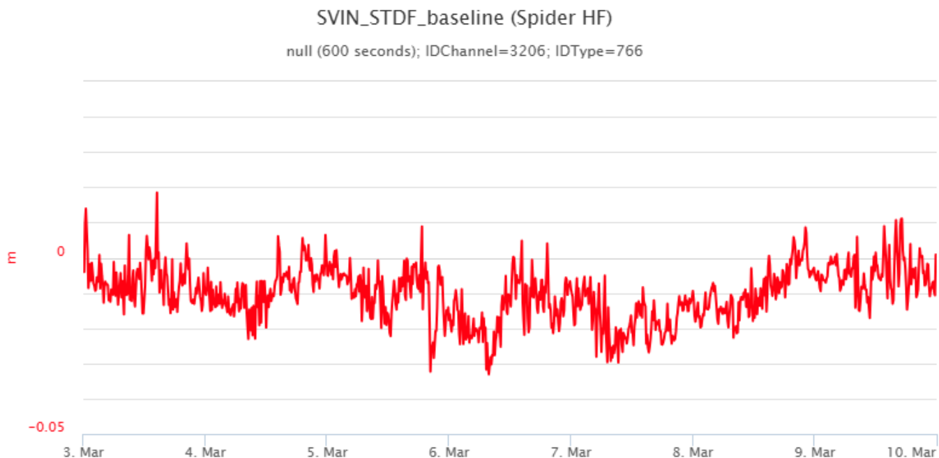
Fig. 5.1 Serie temporale della variazione di distanza tra le stazioni GNSS di San Vincenzo (SVIN) e di Timpone del Fuoco (STDF) nel corso dell'ultima settimana.
