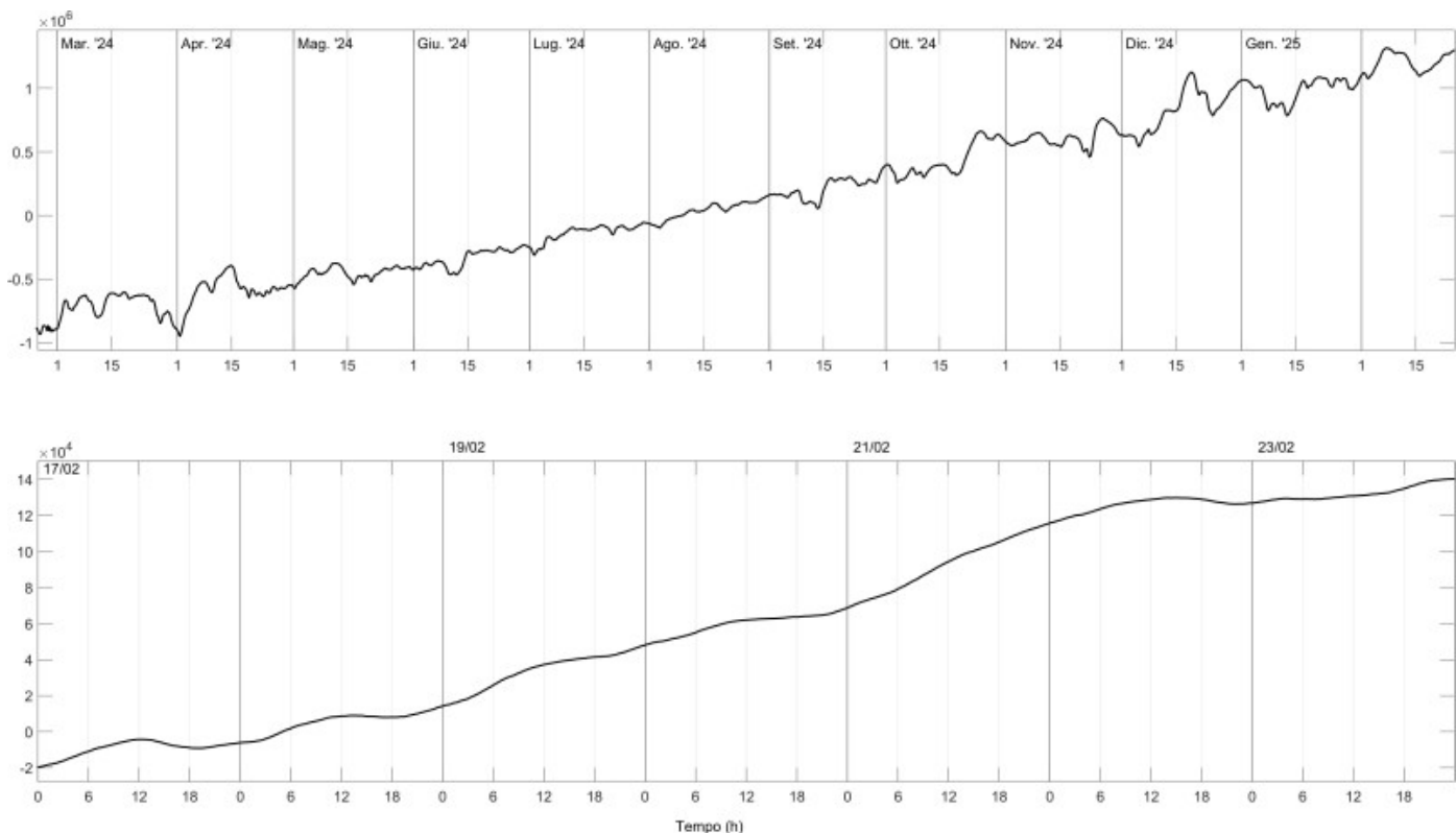
Fig. 4.3 Grafico relativo al dato dilatometrico registrato a SVO: in alto viene mostrato lo strain registrato nell'ultimo anno dal 25/02/2024; in basso quello registrato nell'ultima settimana.
