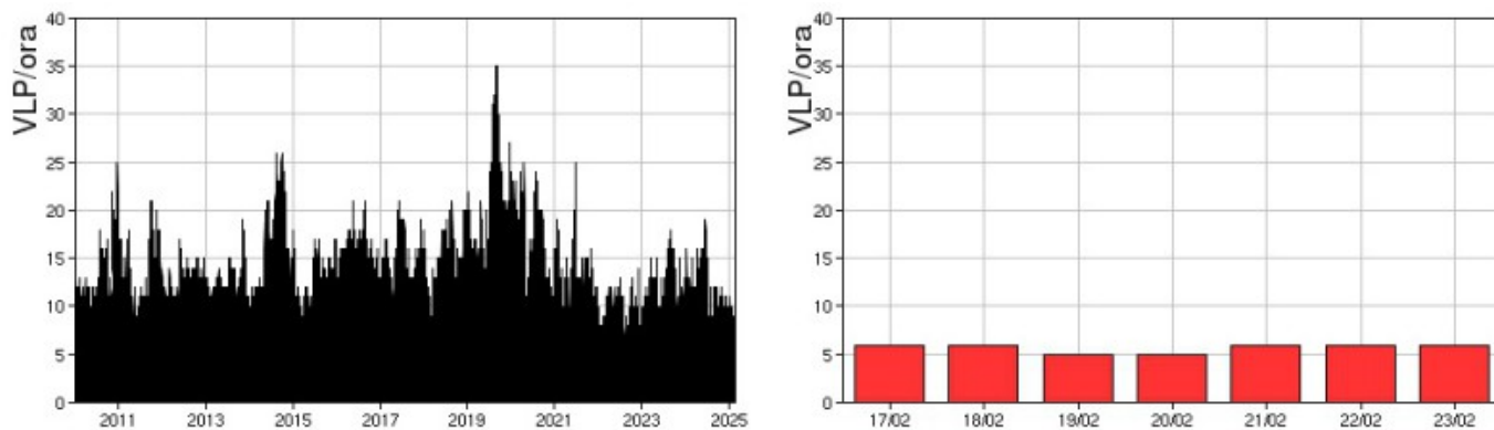
Fig. 4.2 La frequenza di occorrenza dei VLP ha avuto valori compresi tra 5 e 6 eventi/ora.
