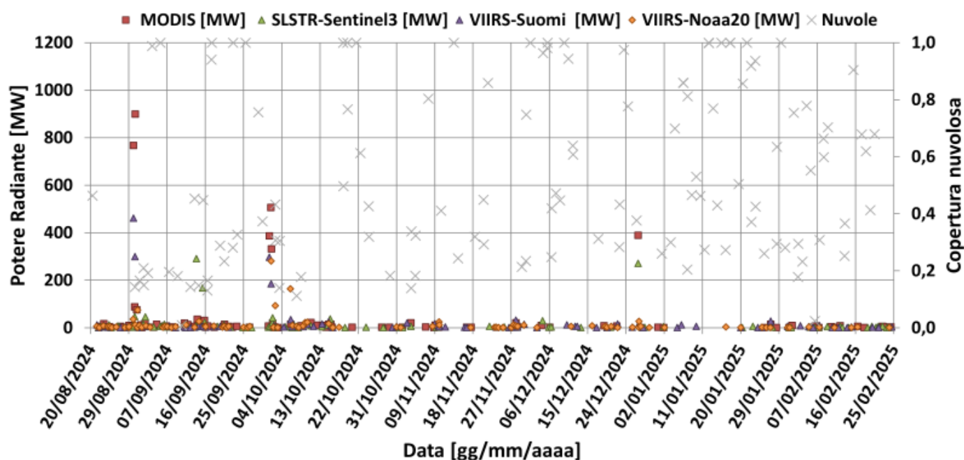
Fig. 7.1 Potere radiante calcolato da dati MODIS (quadrato rosso), SENTINEL-3 SLSTR (triangolo verde) e VIIRS (triangolo viola e rombo giallo) dal 20 agosto 2024 al 25 febbraio 2025.
