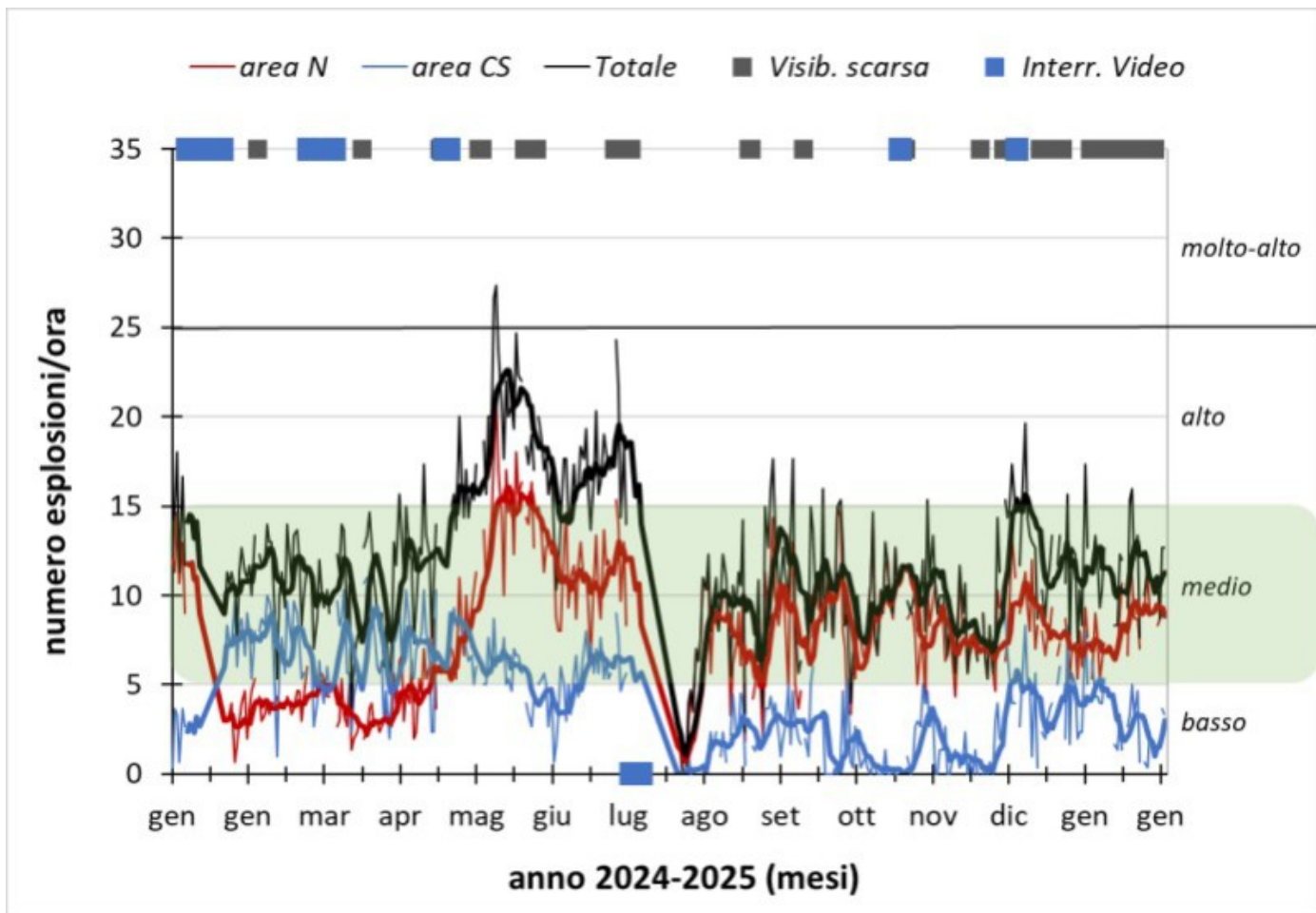
Fig. 3.2 Frequenza media oraria giornaliera e settimanale per area craterica ed in totale dell'attività esplosiva dello Stromboli (rispettivamente linea sottile ed in grassetto). Il top del grafico mostra le condizioni della visibilità, a destra sono riportati i livelli di attività; la fascia verde indica il livello medio tipico dell'attività esplosiva dello Stromboli.
