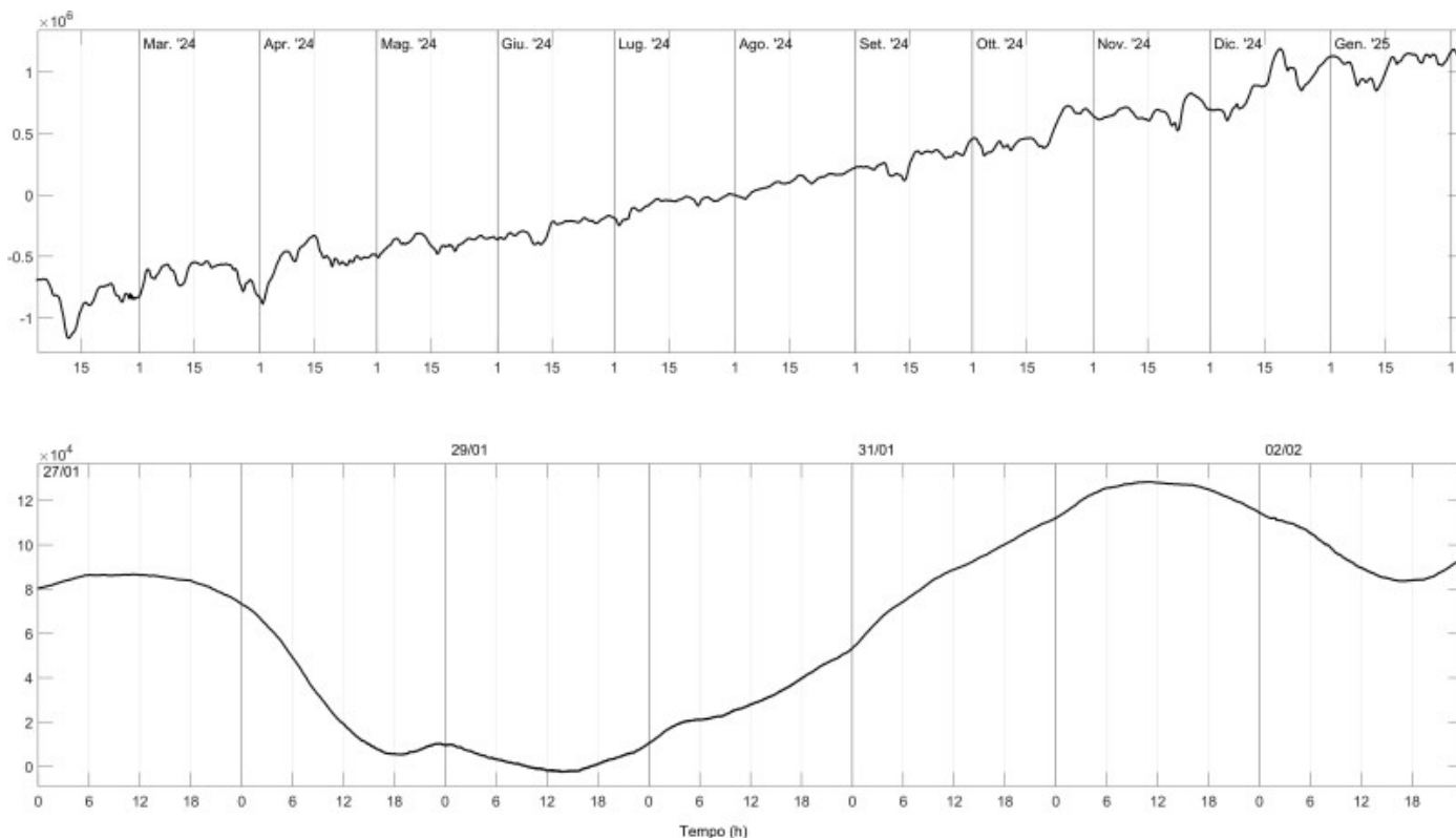
Fig. 4.3 Grafico relativo al dato dilatometrico registrato a SVO: in alto viene mostrato lo strain registrato nell'ultimo anno dal 04/02/2024; in basso quello registrato nell'ultima settimana.
