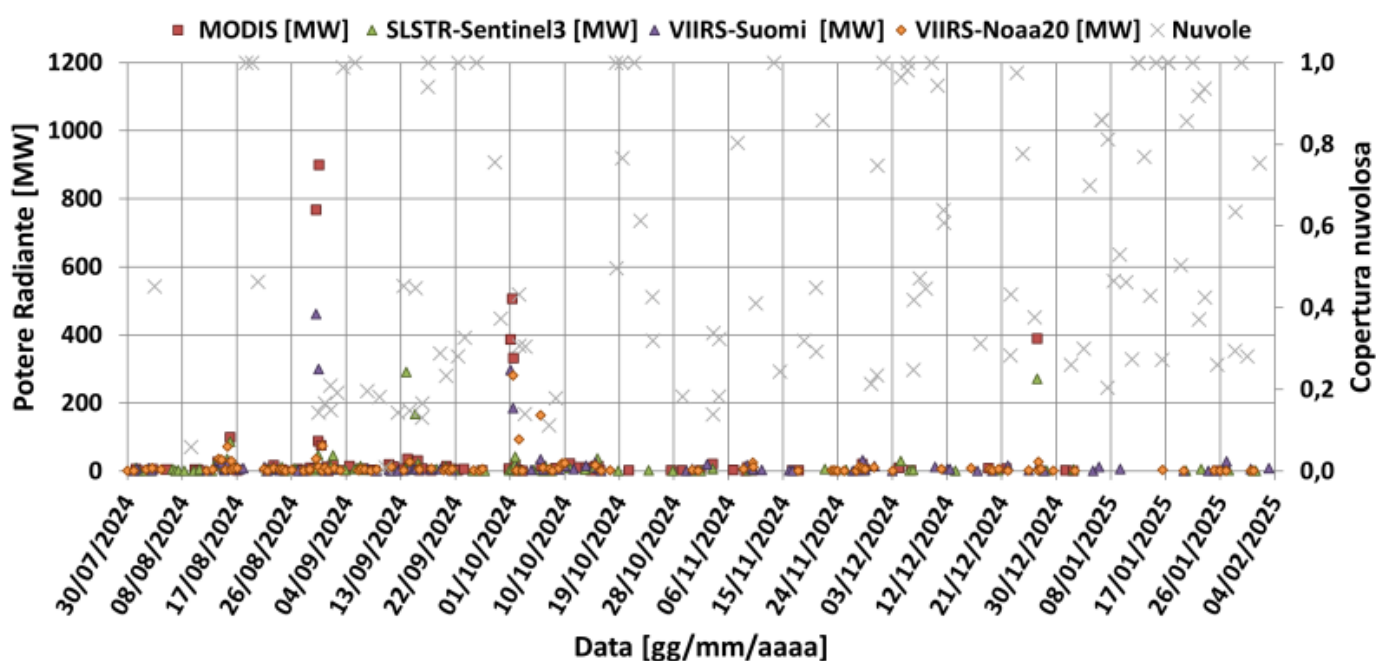
Fig. 7.1 Potere radiante calcolato da dati MODIS (quadrato rosso), SENTINEL-3 SLSTR (triangolo verde) e VIIRS (triangolo viola e rombo giallo) dal 30 luglio 2024 al 4 febbraio 2025.
