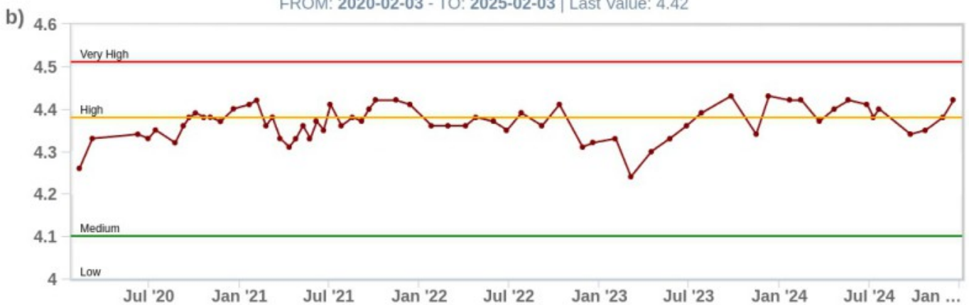
Fig. 6.4 Rapporto isotopico dell'He disciolto nei pozzi termali a) ultimo anno, b) ultimi 5 anni.
