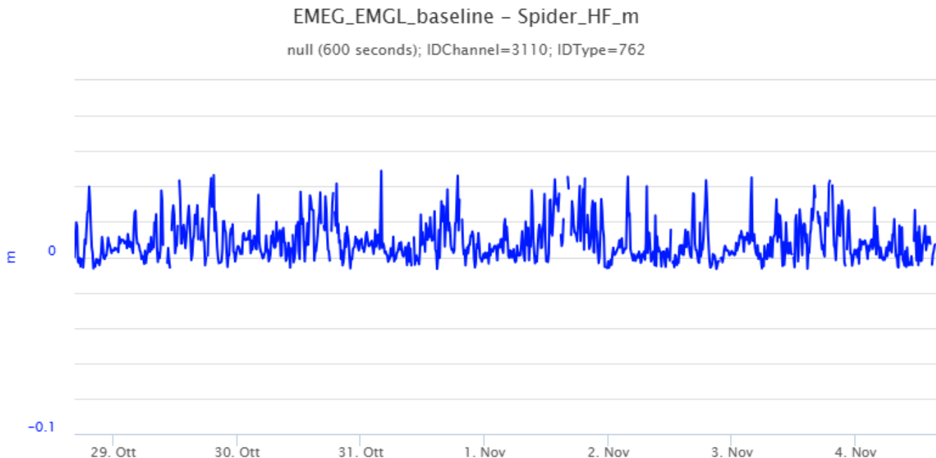
Fig. 6.1 Serie temporale della baseline tra Mt Egitto (EMEG) e Mt Gallo (EMGL) nel corso dell'ultima settimana.
