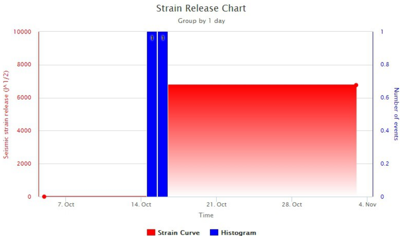
Fig. 4.1 Frequenza giornaliera di accadimento e curva cumulativa del rilascio di strain sismico dei terremoti con M_l pari o
