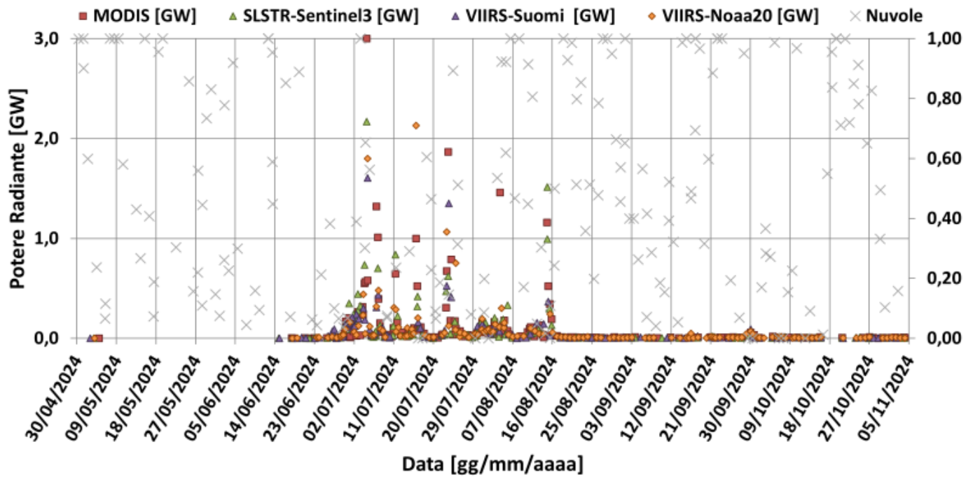
Fig. 8.1 Potere radiante calcolato da dati MODIS (quadrato rosso), SENTINEL-3 SLSTR (triangolo verde) e VIIRS (triangolo viola e rombo giallo) dal 30 aprile 2024 al 5 novembre 2024.
