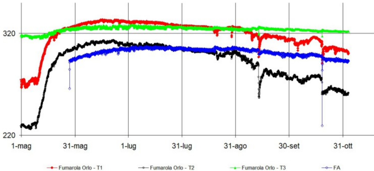
Fig. 3.2 Serie temporale dei valori di temperatura (°C) misurati in continuo nelle fumarole site sull'orlo del versante nord del cono La Fossa (T1 e T2, fumarola F5AT; T3, fumarola F5).
