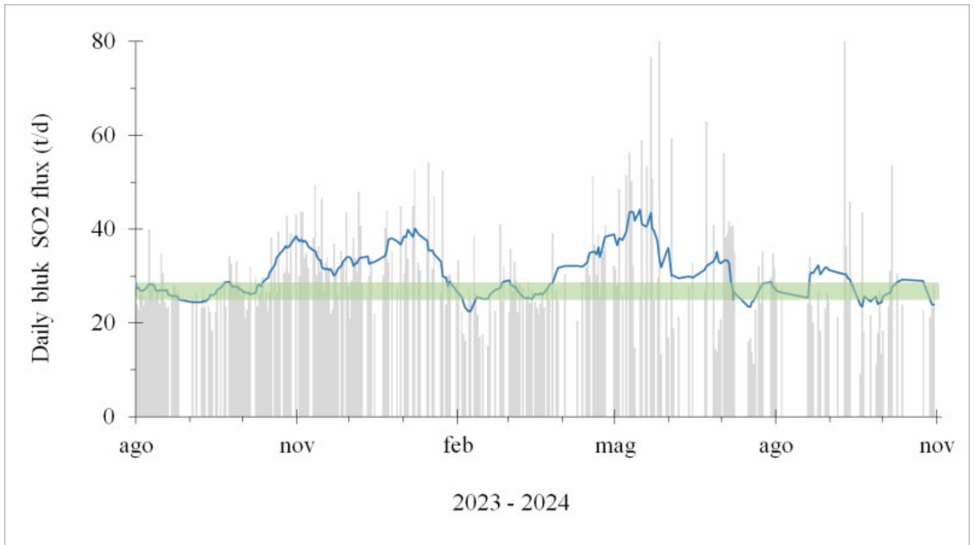
Fig. 5.1 Il flusso di SO 2 medio-giornaliero e medio-settimanale (rispettivamente, barra grigia e linea blu) emesso dal campo fumarolico craterico di Vulcano nel corso dell'ultimo anno.
