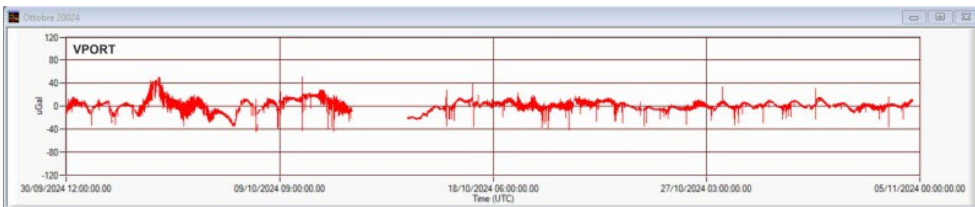
Fig. 13.1 Segnale gravimetrico registrato nella stazione VPORT dalle 12:00 UTC del 30 settembre alle 23:59 UTC del 04 novembre 2024. Il segnale è mediato al minuto. I dati sono corretti per gli effetti della marea terrestre e della deriva strumentale.
