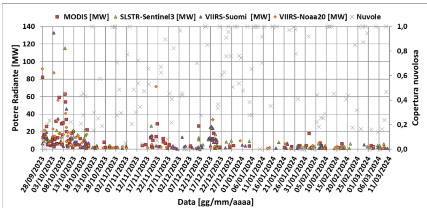
Fig. 7.1 Potere radiante calcolato da dati MODIS (quadrato rosso), SENTINEL-3 SLSTR (triangolo verde) e VIIRS (triangolo viola e rombo giallo) dal 28 settembre 2023 al 11 marzo 2024. Per l'intero periodo analizzato è anche riportato l'indice di nuvolosità.
