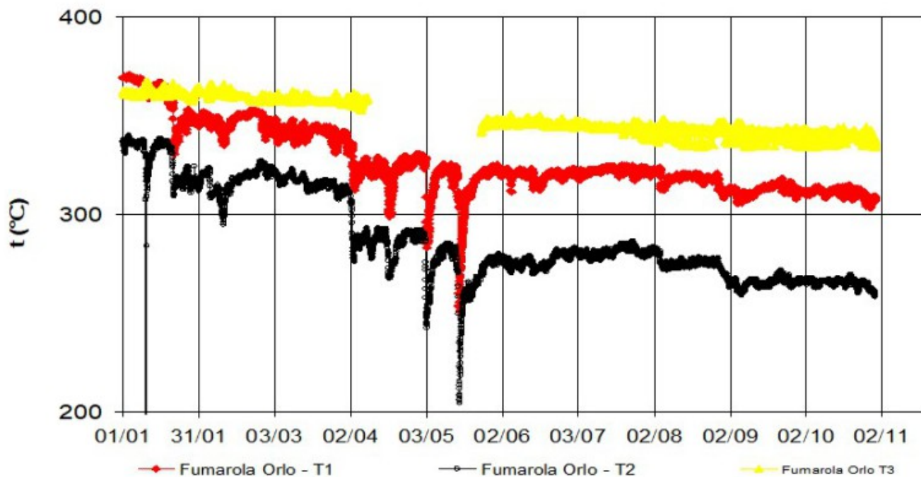
Fig. 3.2 Serie temporale dei valori di temperatura (°C) misurati in continuo nelle fumarole poste sull'orlo del versante nord del cono La Fossa (fumarola F5AT, segnali T1 in rosso e T2 in nero; fumarola F5, segnale T3 in giallo).
