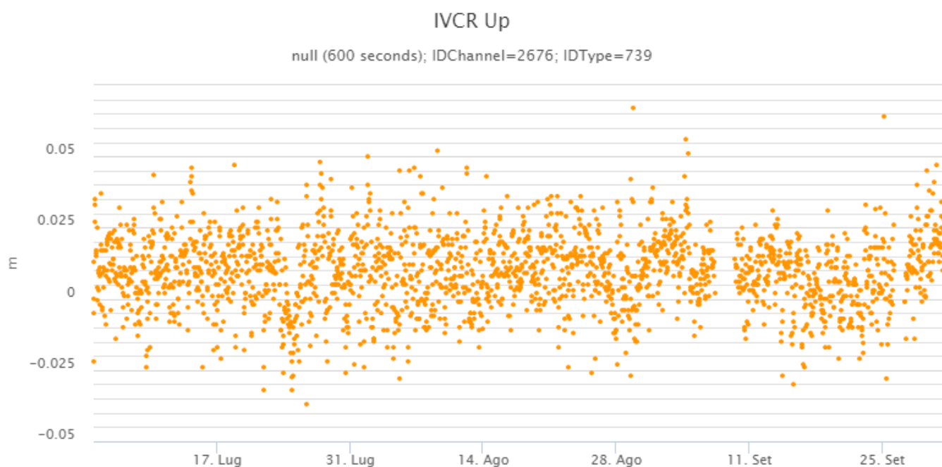
Fig. 11.1 Serie temporale della variazione della componente verticale (verso positivo, in sollevamento) della stazione di Vulcano Cratere (IVCR) nel corso dell'ultimo trimestre.
