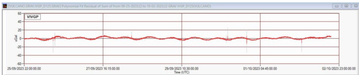
Fig. 13.1 Segnale gravimetrico registrato nella stazione VVIGP dalle 22:00 UTC del 25 settembre alle 23:00 UTC del 02 ottobre 2023. In grigio segnale acquisito al secondo; in rosso il segnale mediato al minuto. I dati sono corretti per gli effetti della marea terrestre e della deriva strumentale.
