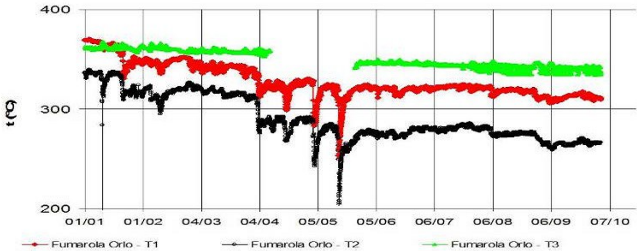
Fig. 3.2 Serie temporale dei valori di temperatura ( ^{\circ}\text{C} ) misurati in continuo nelle fumarole poste sull'orlo del versante nord del cono La Fossa (fumarola F5AT, segnali T1 in rosso e T2 in nero; fumarola F5, segnale T3 in verde).
