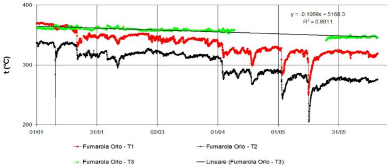
Fig. 3.2 Serie temporale dei valori di temperatura (°C) misurati in continuo nelle fumarole poste sull'orlo del versante nord del cono La Fossa (fumarola F5AT, segnali T1 in rosso e T2 in nero; fumarola F5, segnale T3 in verde).
