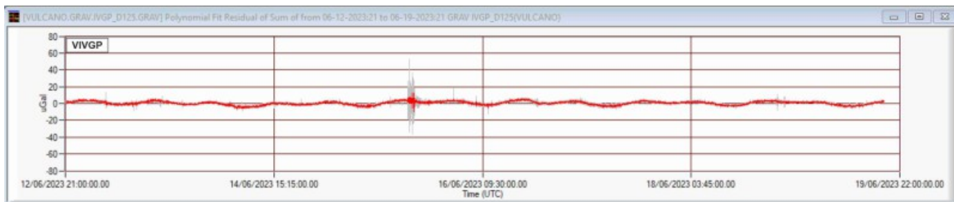
Fig. 13.1 Segnale gravimetrico registrato nella stazione VVIGP dalle 21:00 UTC del 12 alle 21:00 UTC del 19 giugno 2023. In grigio segnale acquisito al secondo; in rosso il segnale mediato al minuto. I dati sono corretti per gli effetti della marea terrestre e della deriva strumentale.
