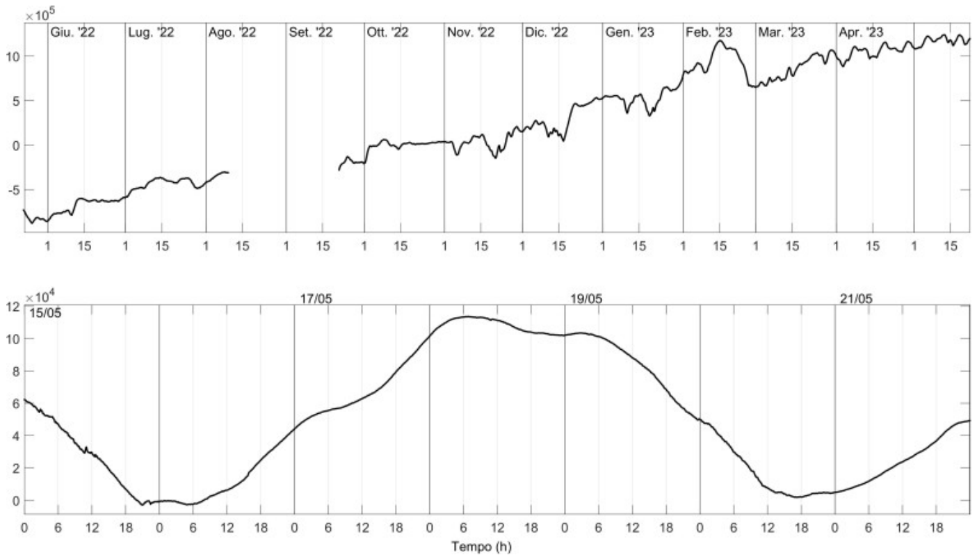
Fig. 4.3 Grafico relativo al dato dilatometrico registrato a SVO: in alto viene mostrato lo strain registrato dal 23/05/2022, in basso quello nell'ultima settimana.
