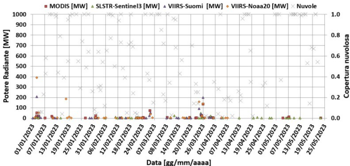
Fig. 7.1 Potere radiante calcolato da dati MODIS (quadrato rosso), SENTINEL-3 (triangolo verde) e VIIRS (triangolo viola e rombo giallo) dal primo gennaio alla sera del 22 maggio 2023. Per l'intero periodo analizzato è anche riportato l'indice di nuvolosità.
