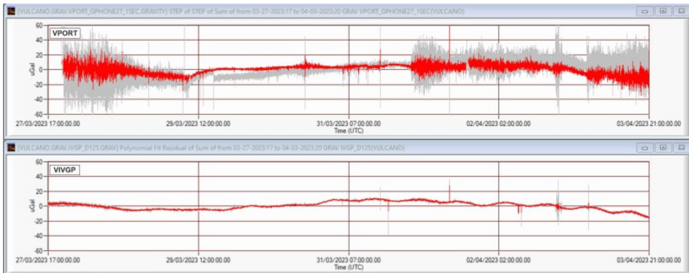
Fig. 13.1 Segnali gravimetrici registrati nelle stazioni VPORT (in alto) e VIVGP (in basso) dalle 17:00 UTC del 27 marzo alle 20:00 UTC del 03 aprile 2023. In grigio segnali acquisiti al secondo; in rosso i segnali mediati al minuto. I dati sono corretti per gli effetti della marea terrestre e della deriva strumentale.
