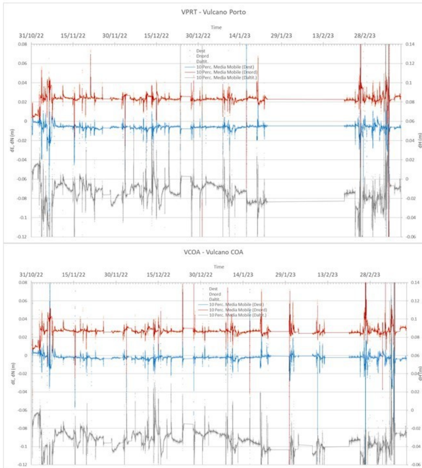
Fig. 14.1 Spostamenti misurati alle stazioni GNSS mobili del COA e di Vulcano Porto dall'inizio del mese di novembre 2022. La linea continua rappresenta una media mobile su una finestra di 10 minuti.
