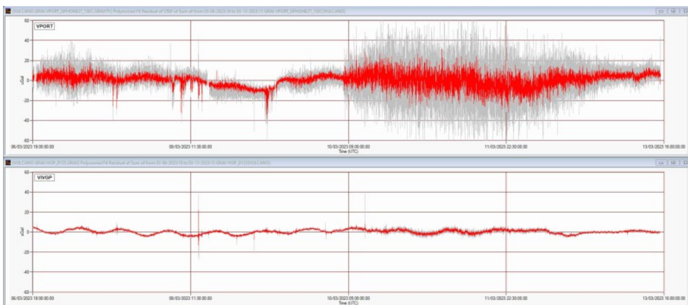
Fig. 13.1 Segnali gravimetrici registrati nelle stazioni VPORT (in alto) e VIVGP (in basso) dalle 18:00 UTC del 06 marzo alle 16:00 UTC del 13 marzo 2023. In grigio segnali acquisiti al secondo; in rosso i segnali mediati al minuto. I dati sono corretti per gli effetti della marea terrestre e della deriva strumentale.
