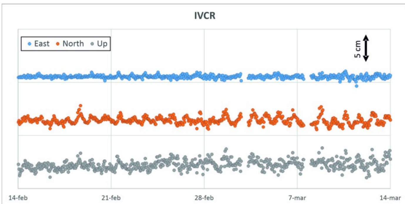
Fig. 11.1 Serie temporale delle componenti Est, Nord e Verticale della stazione di Vulcano Cratere (IVCR) nel corso dell'ultimo mese
