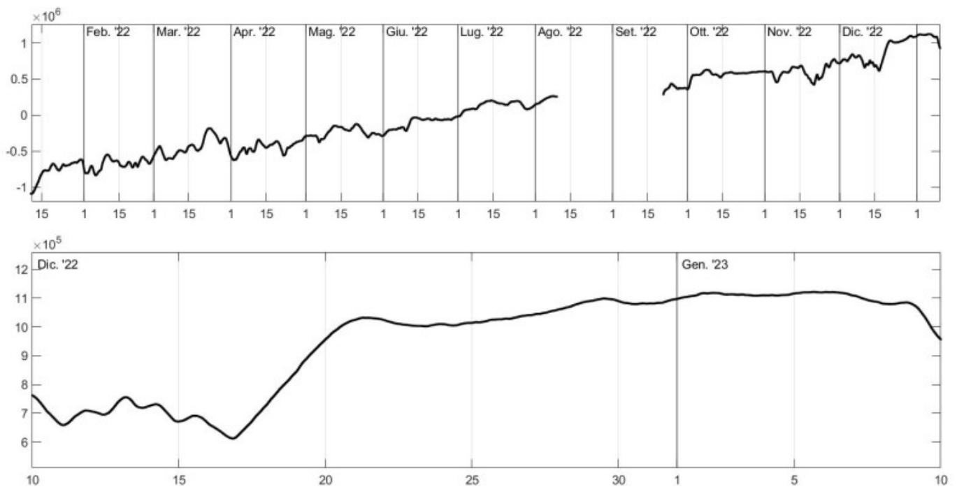
Fig. 4.3 Grafico relativo al dato dilatometrico registrato a SVO: in alto viene mostrato lo strain registrato dal 10/01/2022, in basso quello nell'ultima settimana.
