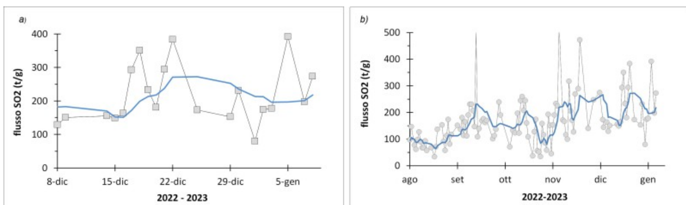
Fig. 6.1 Flusso di SO 2 medio-giornaliero nel corso degli ultimi mesi (a) e dell'ultimo semestre (b)
