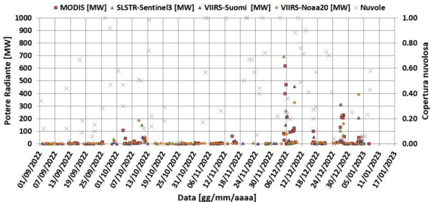
Fig. 7.1 Potere radiante calcolato da dati MODIS (quadrato rosso), SENTINEL-3 (triangolo verde) e VIIRS (triangolo viola e rombo giallo) dal primo settembre 2022 alla mattina del 9 gennaio 2023. Per l'intero periodo analizzato è anche riportato l'indice di nuvolosità.
