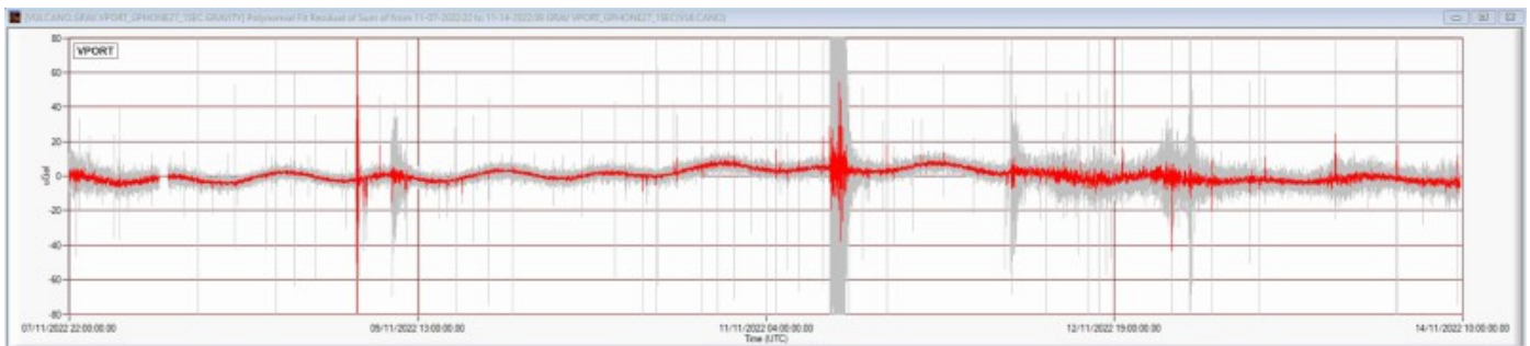
Fig. 13.1 Segnale gravimetrico registrato nella stazione VPORT dalle 22:00 UTC del 07 alle 10:00 UTC del 14 novembre 2022. In grigio il segnale acquisito al secondo; in rosso il segnale mediato al minuto. I segnali sono corretti per gli effetti della marea terrestre e della deriva strumentale.
