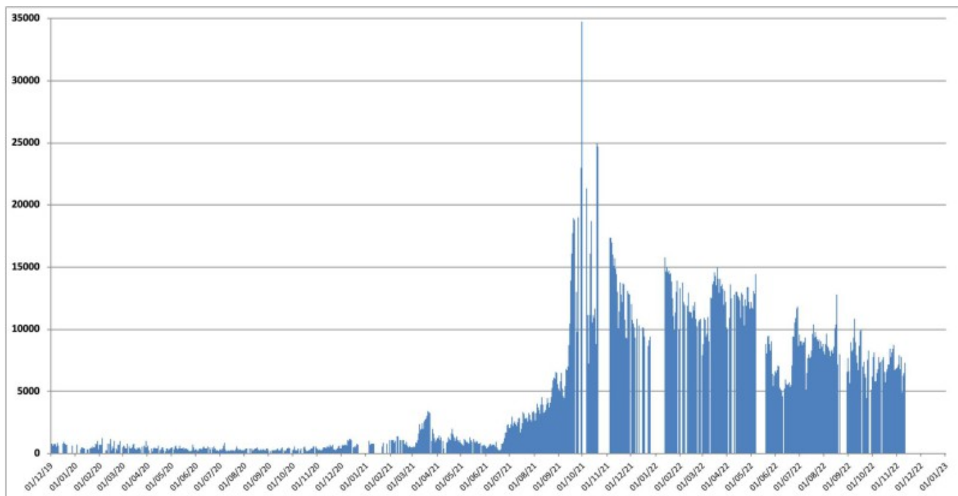
Fig. 4.1 Registrazione automatica del flusso diffuso di CO2 dal suolo nel sito posto a Est dell'area fumarolica (sito VSCS).
