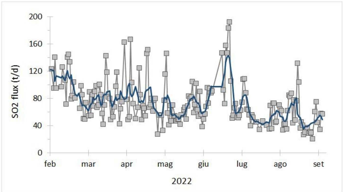
Fig. 5.1 Flusso di SO 2 medio-giornaliero e medio-settimanale (rispettivamente, curva nera e blu) emesso dal campo fumarolico craterico di Vulcano nell'ultimo semestre.
