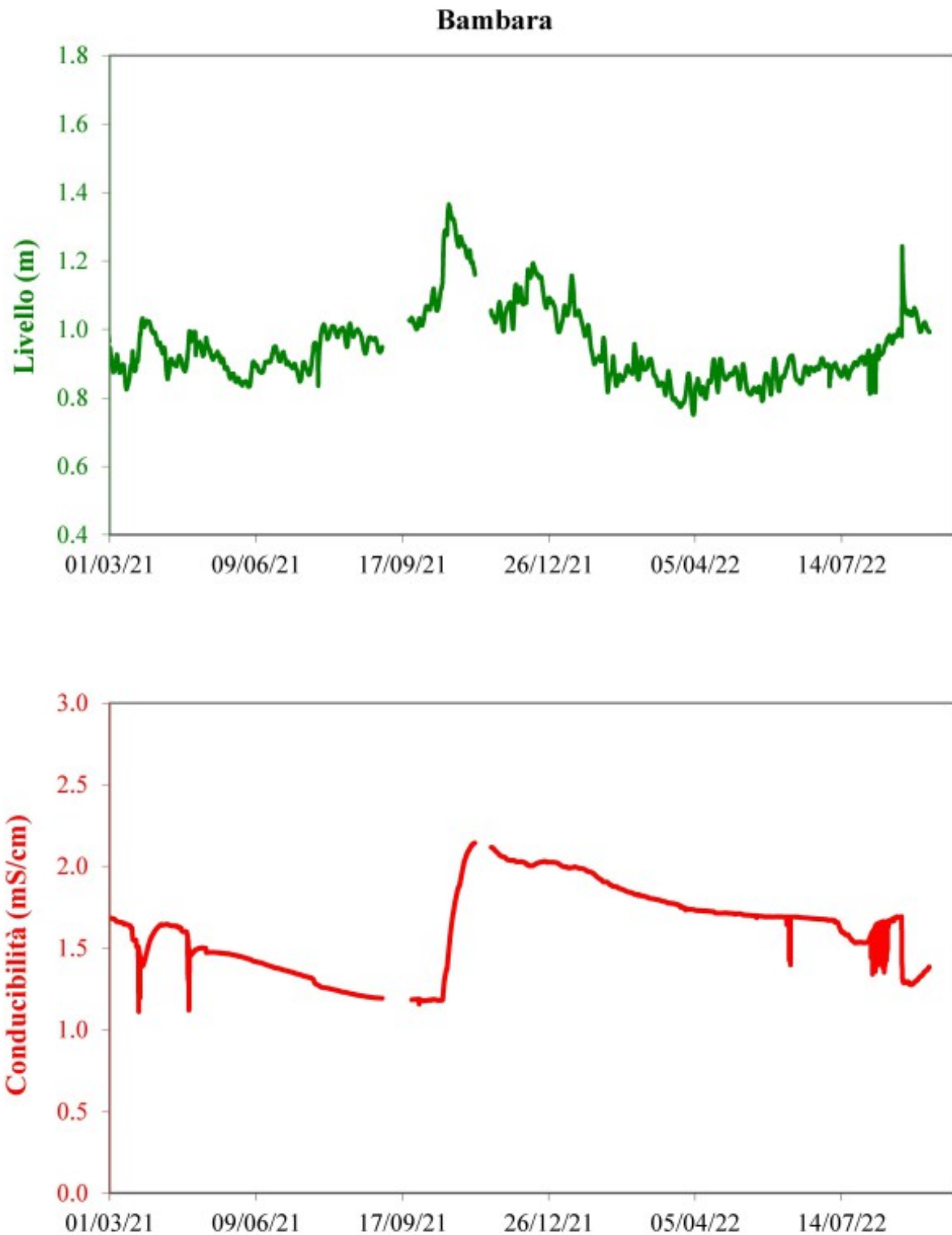
Fig. 8.2 Dati di livello freatico e di conducibilità riportata a 20°C, acquisiti in automatico nel pozzo Bambara.
