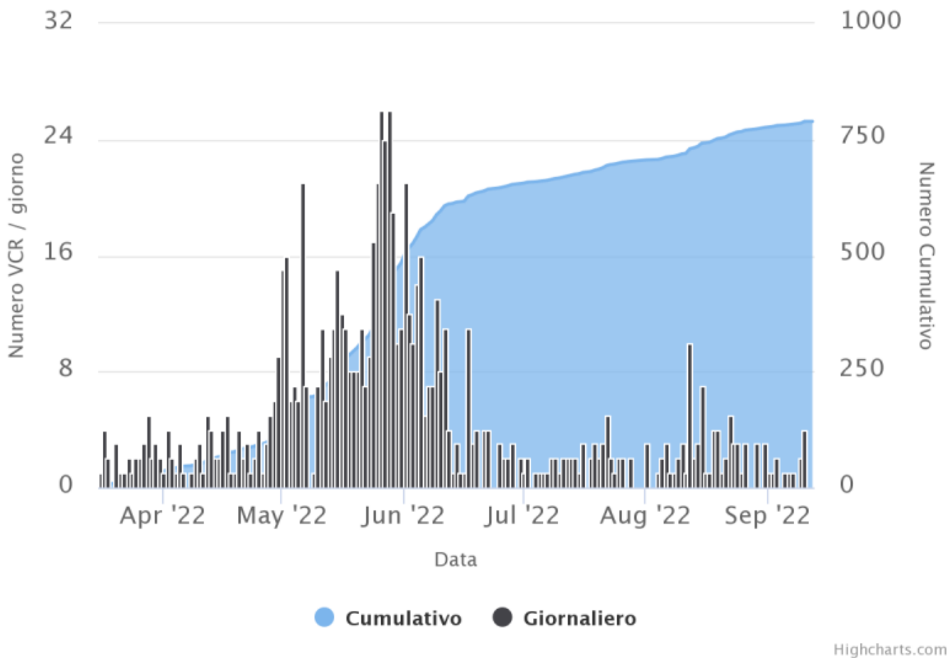
Fig. 9.1 1 Frequenza giornaliera e numero cumulativo delle micrososse (frequenza di picco tra 1 e 30 Hz) che caratterizzano la sismicità locale di Vulcano negli ultimi 180 giorni.
