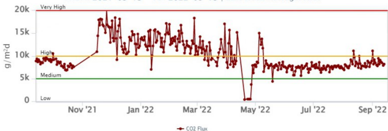
Fig. 6.2 Andamento temporale del flusso di CO 2 dal suolo in area sommitale (stazione STR02): a) ultimi tre mesi; b) ultimo anno
