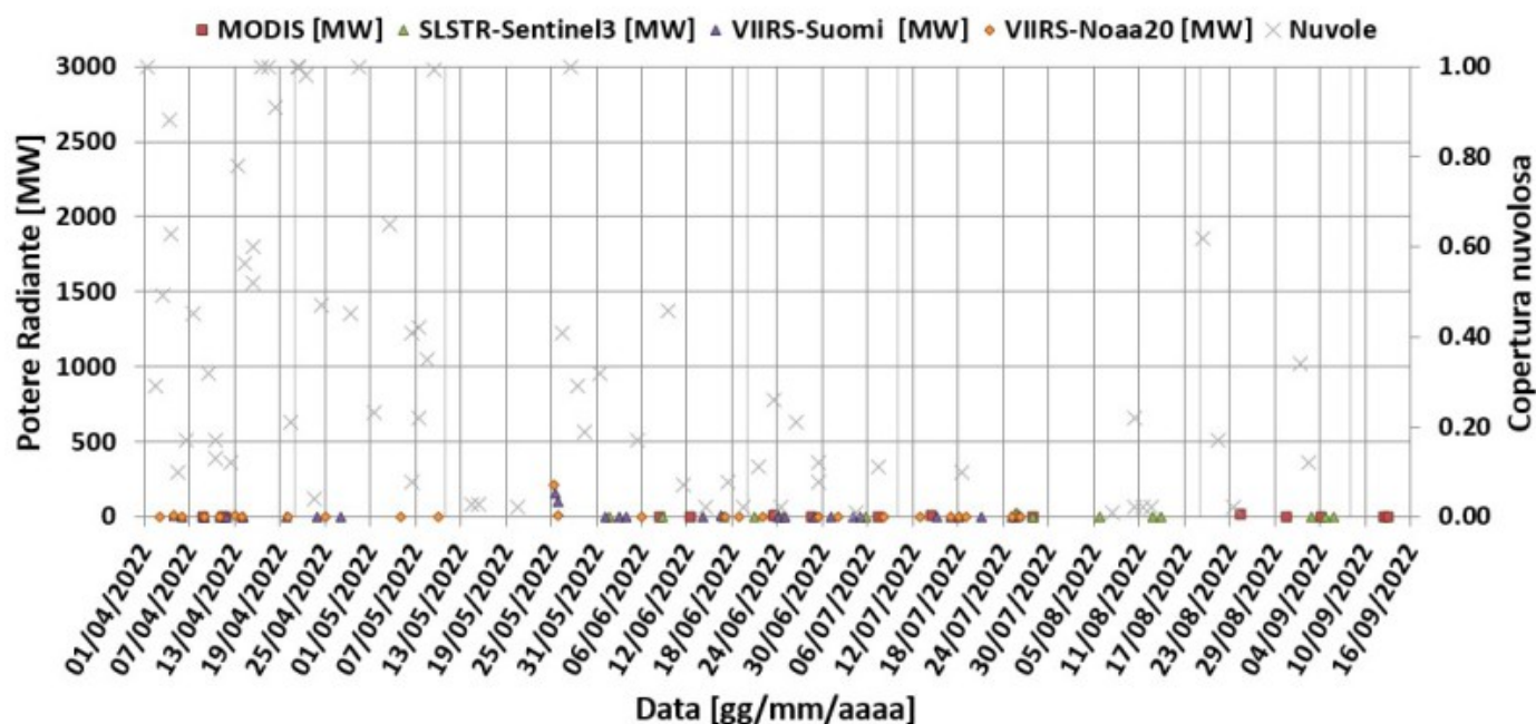
Fig. 7.1 Potere radiante calcolato da dati MODIS (quadrato rosso), SENTINEL-3 (triangolo verde) e VIIRS (triangolo viola e rombo giallo) dal primo aprile al 12 settembre 2022. Per l'intero periodo analizzato è anche riportato l'indice di nuvolosità.
