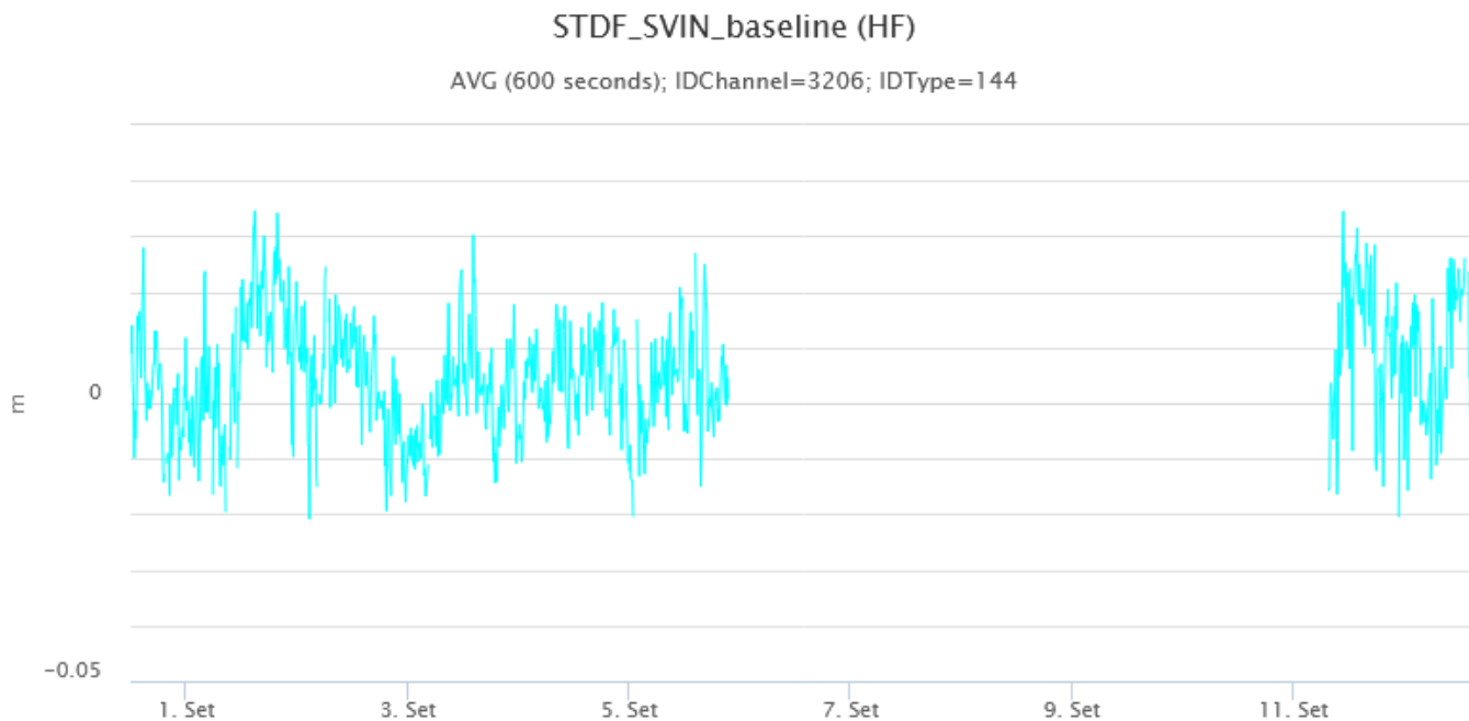
Fig. 5.1 Serie temporale della variazione di distanza tra le stazioni GNSS di STDF e di SVIN a partire dal 1 settembre.
