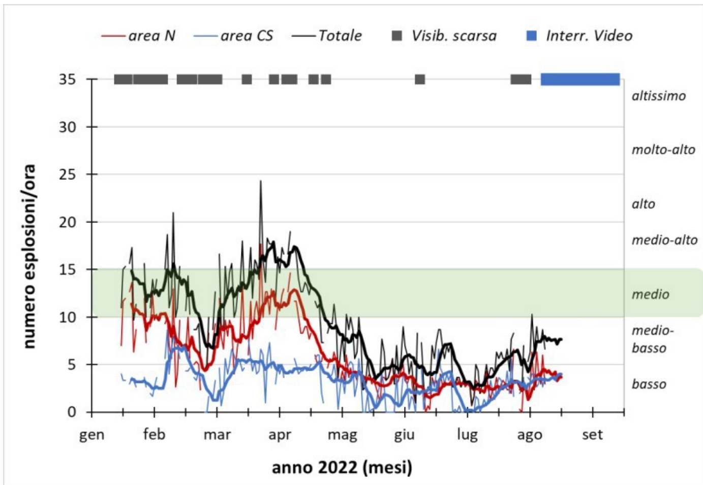
Fig. 3.3 Fig. 3.3 Frequenza media oraria giornaliera e settimanale per area craterica ed in totale dell'attività esplosiva dello Stromboli (rispettivamente linea sottile ed in grassetto). Al top del grafico è riportata la condizioni di osservazione del dato e a destra i livelli di attività; la barra verde indica il livello medio tipico dell'attività esplosiva dello Stromboli. Dato aggiornato al 14/08/22 causa l'indisponibilità dei segnali video in seguito al danneggiamento della fibra ottica il 12 agosto
