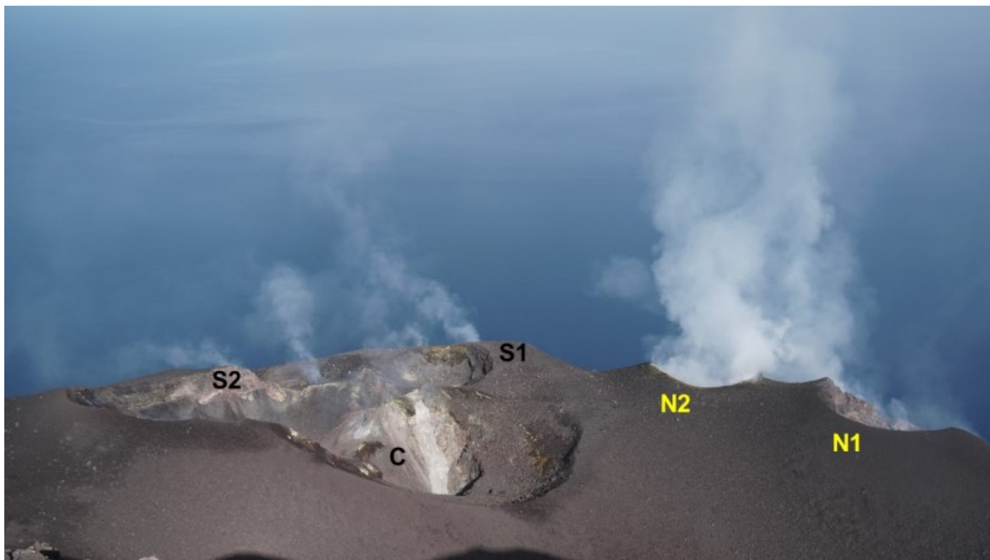
Fig. 3.1 Foto della terrazza craterica effettuata dal Pizzo sopra la fossa con l'ubicazione dei settori craterici delle due aree crateriche (N e CS)
