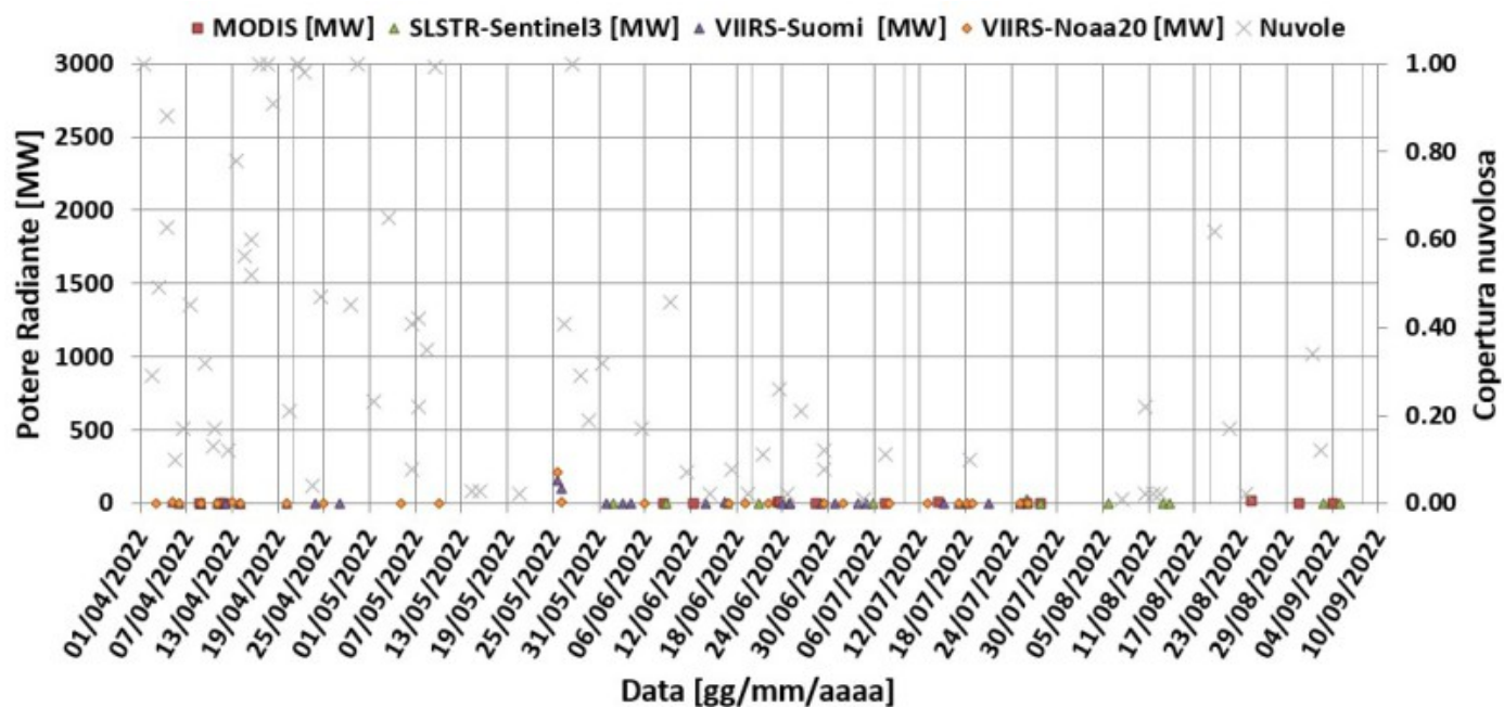
Fig. 7.1 Potere radiante calcolato da dati MODIS (quadrato rosso), SENTINEL-3 (triangolo verde) e VIIRS (triangolo viola e rombo giallo) dal primo aprile al 4 settembre 2022. Per l'intero periodo analizzato è anche riportato l'indice di nuvolosità.
