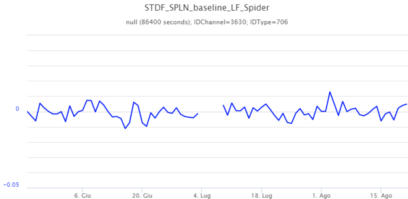
Fig. 5.1 Serie temporale della variazione di distanza tra le stazioni GNSS di STDF e di SPLN, nel corso degli ultimi 3 mesi.
