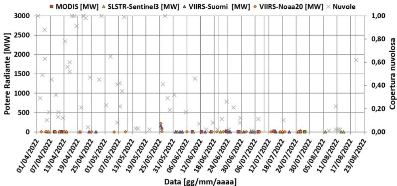
Fig. 7.1 Potere radiante calcolato da dati MODIS (quadrato rosso), SENTINEL-3 (triangolo verde) e VIIRS (triangolo viola e rombo giallo) dal primo aprile al 21 agosto 2022. Per l'intero periodo analizzato è anche riportato l'indice di nuvolosità.
