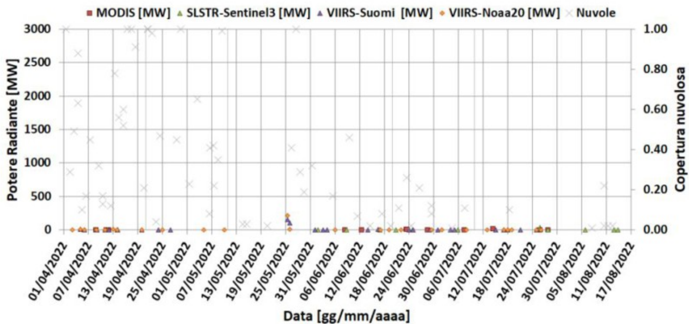
Fig. 7.1 Potere radiante calcolato da dati MODIS (quadrato rosso), SENTINEL-3 (triangolo verde) e VIIRS (triangolo viola e rombo giallo) dal primo aprile al 16 agosto 2022. Per l'intero periodo analizzato è anche riportato l'indice di nuvolosità.
