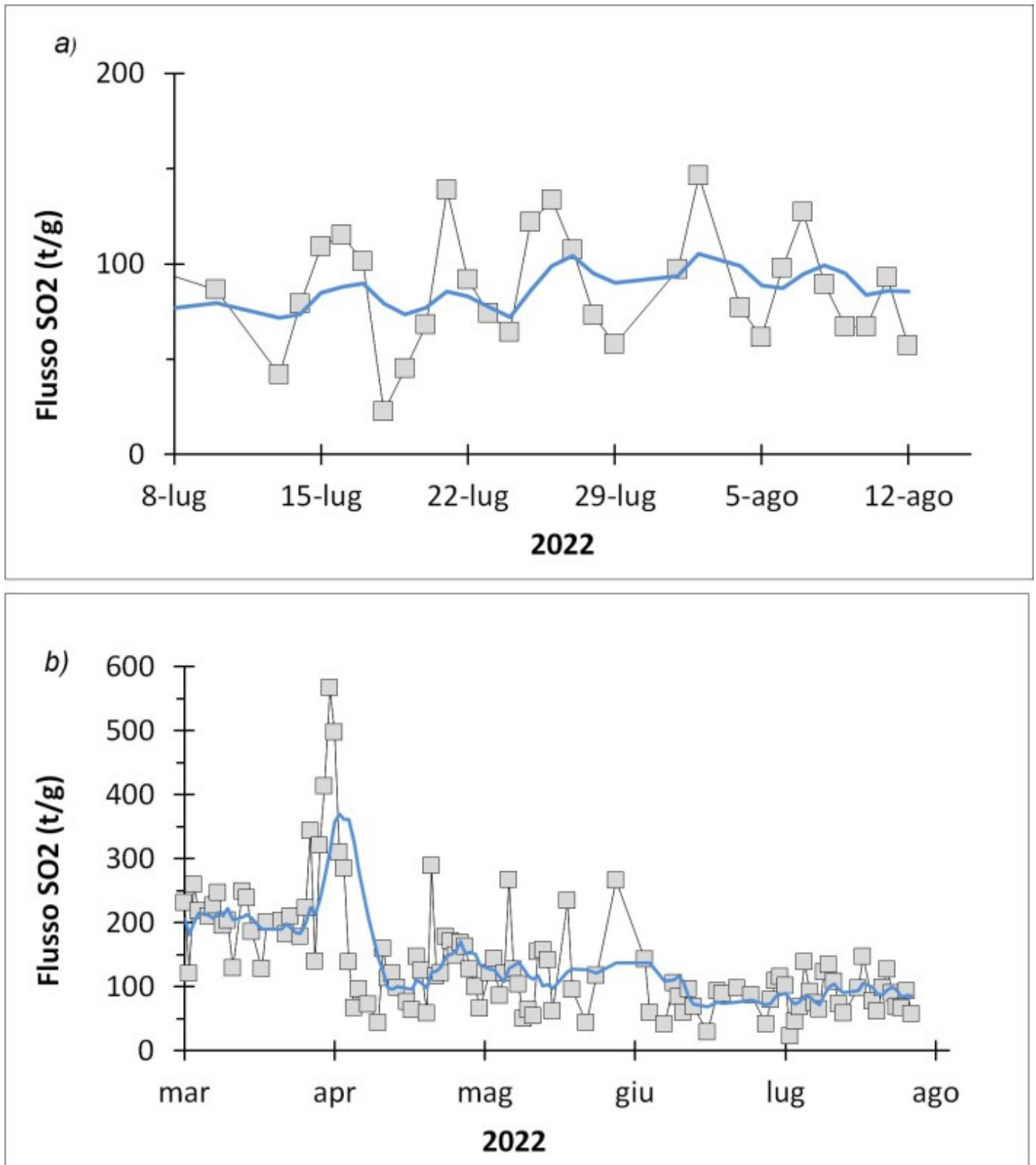
Fig. 6.1 Flusso di SO 2 medio-giornaliero nel corso dell'ultimo mese (a) e dell'ultimo semestre (b)
