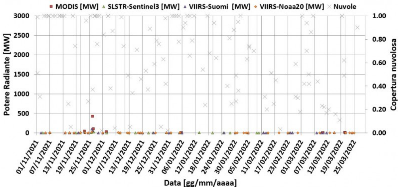
Fig. 7.1 Potere radiante calcolato da dati MODIS (quadrato rosso), SENTINEL-3 (triangolo verde) e VIIRS (triangolo viola e rombo giallo) dal primo novembre 2021 al 27 marzo 2022. Per l'intero periodo analizzato è anche riportato l'indice di nuvolosità.
