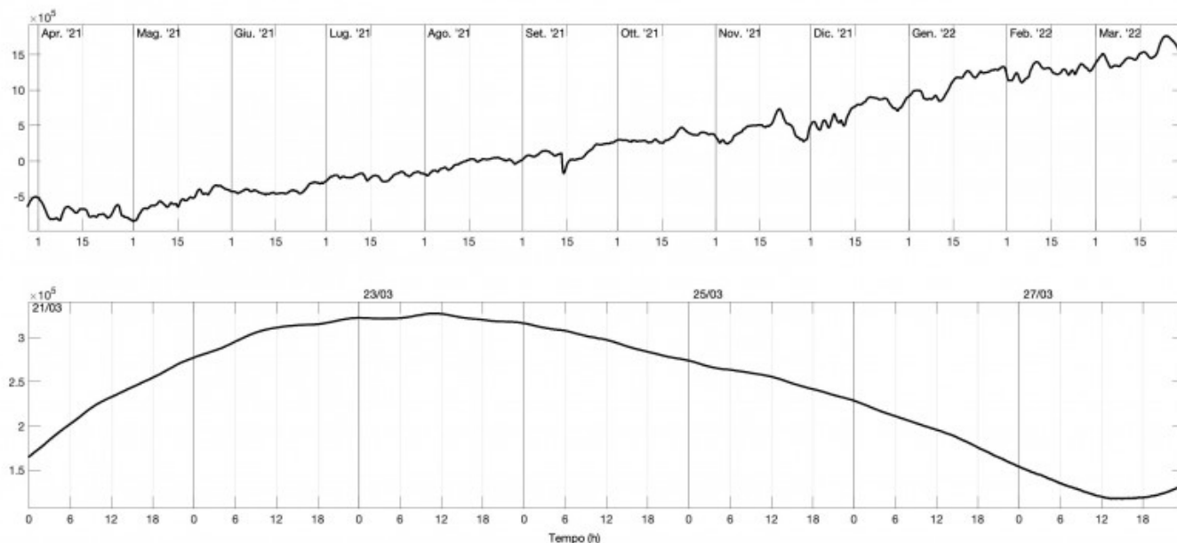
Fig. 4.4 Grafico relativo al dato dilatometrico registrato a SVO: in alto viene mostrato lo strain registrato dal 29/03/2021, in basso quello nell'ultima settimana.
