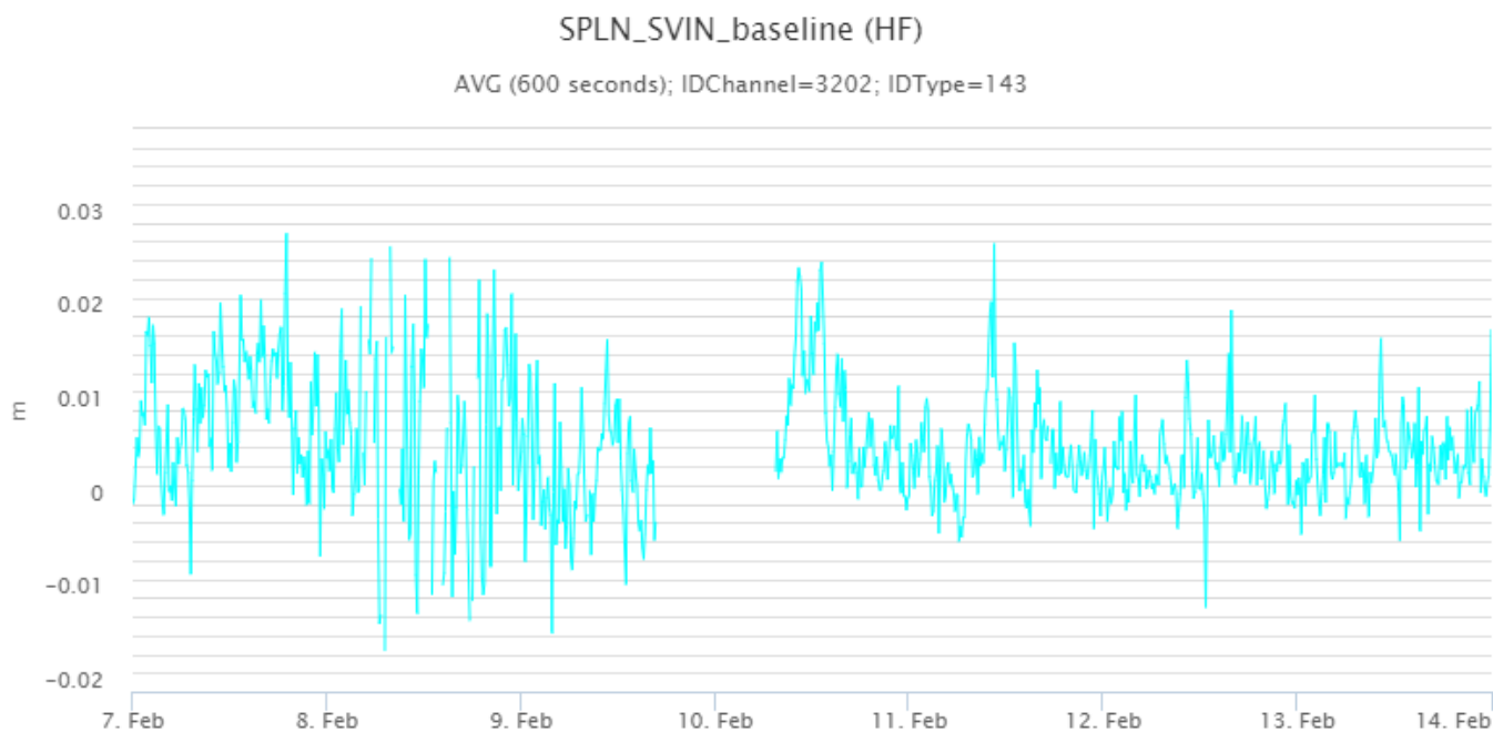
Fig. 5.2 Variazione di distanza Punta Lena (SPLN) - San Vincenzo (SVIN)
