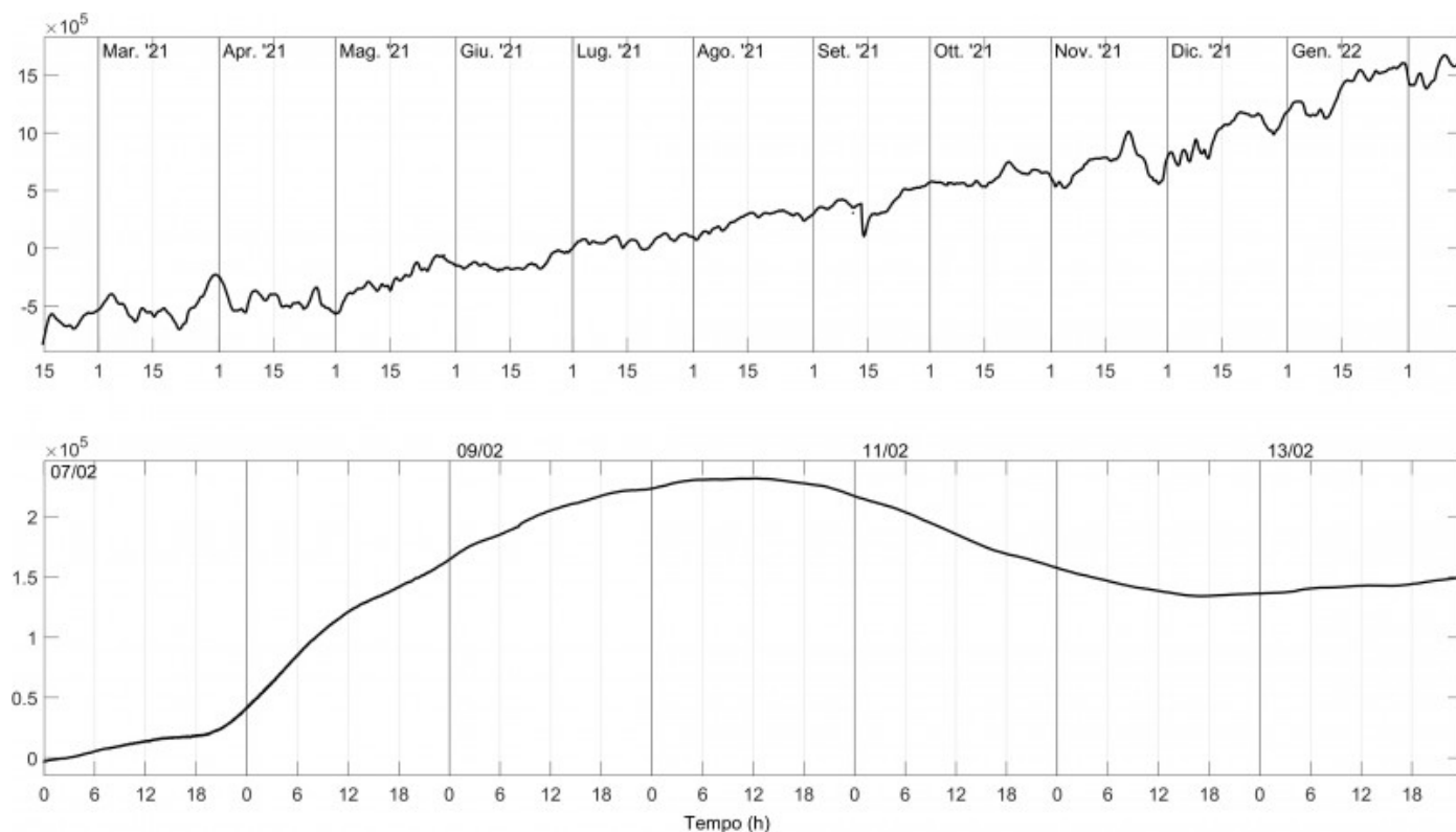
Fig. 4.4 Grafico relativo al dato dilatometrico registrato a SVO: in alto viene mostrato lo strain registrato dal 08/02/2021, in basso quello nell'ultima settimana.
