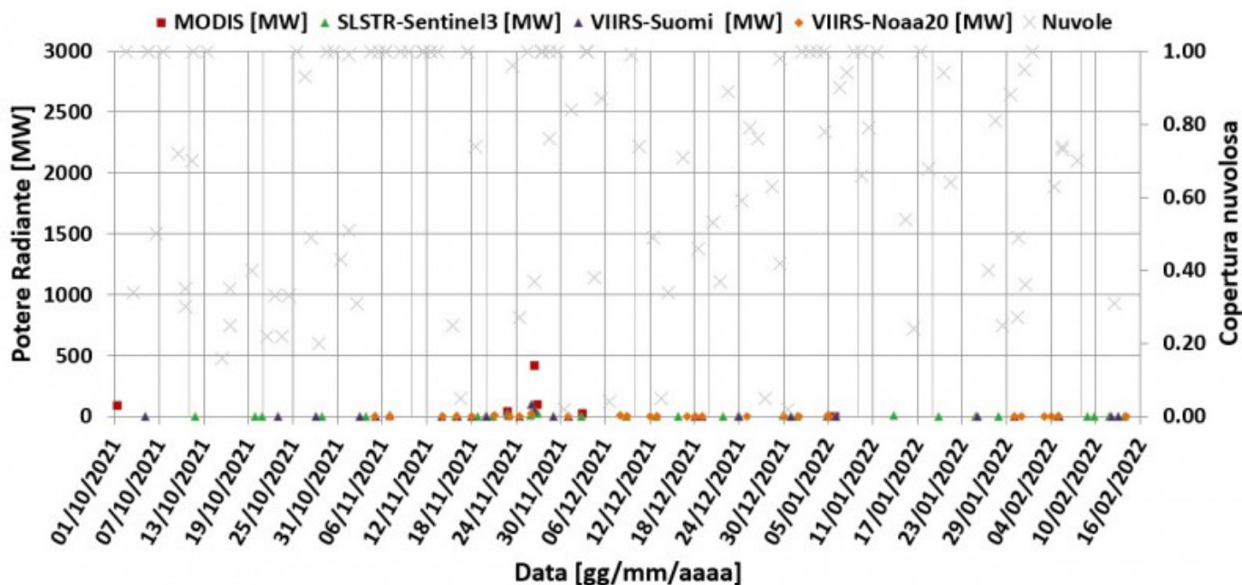
Fig. 7.1 Potere radiante calcolato da dati MODIS (quadrato rosso), SENTINEL-3 (triangolo verde) e VIIRS (triangolo viola e rombo giallo) dal primo ottobre 2021 al 13 febbraio 2022. Per l'intero periodo analizzato è anche riportato l'indice di nuvolosità.
