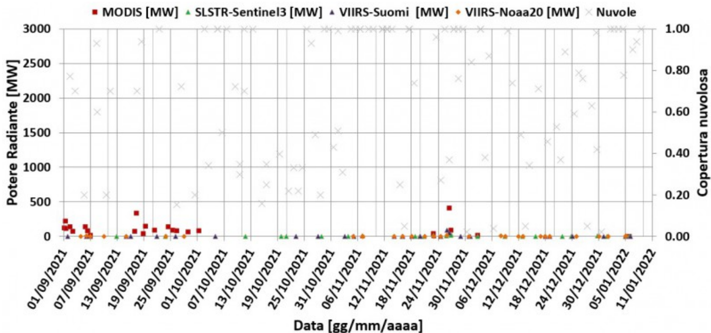
Fig. 7.1 Potere radiante calcolato da dati MODIS (quadrato rosso), SENTINEL-3 (triangolo verde) e VIIRS (triangolo viola e rombo giallo) dal primo settembre 2021 al 9 gennaio 2022. Per l'intero periodo analizzato è anche riportato l'indice di nuvolosità.
