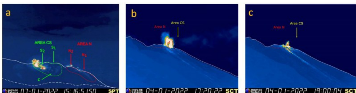
Fig. 3.2 Attività esplosiva dello Stromboli monitorata attraverso la telecamera di sorveglianza dell'INGV-OE posta Pizzo (a) e a quota 190 (b e c).
