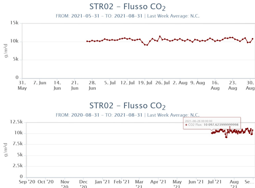
Fig. 6.2 - Andamento temporale del flusso di CO 2 dai suoli: a) ultimi tre mesi; b) ultimo anno. Data ripristino: 24 giugno 2021.
