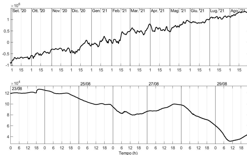
Fig. 4.4 - Grafico relativo al dato dilatometrico registrato a SVO: in alto viene mostrato lo strain registrato dal 23/08/2020, in basso quello nell'ultima settimana.
