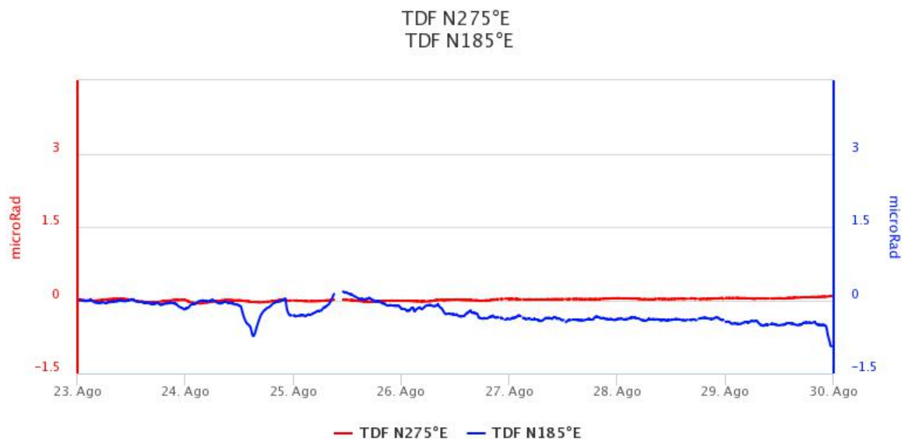
Fig. 5.2 - Serie temporale delle componenti N275E e N185E della stazione clinometrica di TDF nel corso dell'ultima settimana (microrad).
