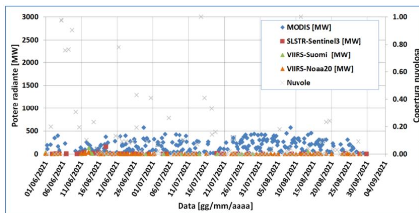
Fig. 7.1 - Potere radiante calcolato da dati MODIS (rombo blu), SENTINEL-3 (quadrato rosso) e VIIRS (triangolo arancione e triangolo verde) dal primo giugno al 30 agosto 2021. Per l'intero periodo analizzato è anche riportato l'indice di nuvolosità.
