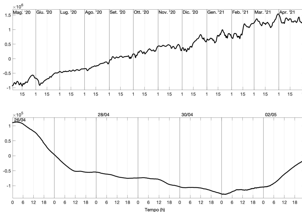
Fig. 4.4 - Grafico relativo al dato dilatometrico registrato a SVO: in alto viene mostrato lo strain registrato dal 03/05/2020, in basso quello nell'ultima settimana.
