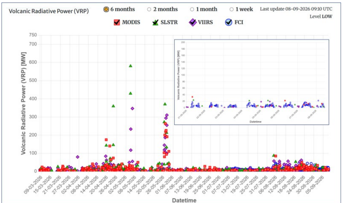
Fig. 7.2 Potere radiante calcolato da dati MODIS (quadrato rosso), SENTINEL-3 SLSTR (triangolo verde), VIIRS (triangolo viola e rombo giallo), MTG-FCI (triangolo blu) e copertura nuvolosa ("x" grigia) dal 3 marzo 2026 all'8 settembre
