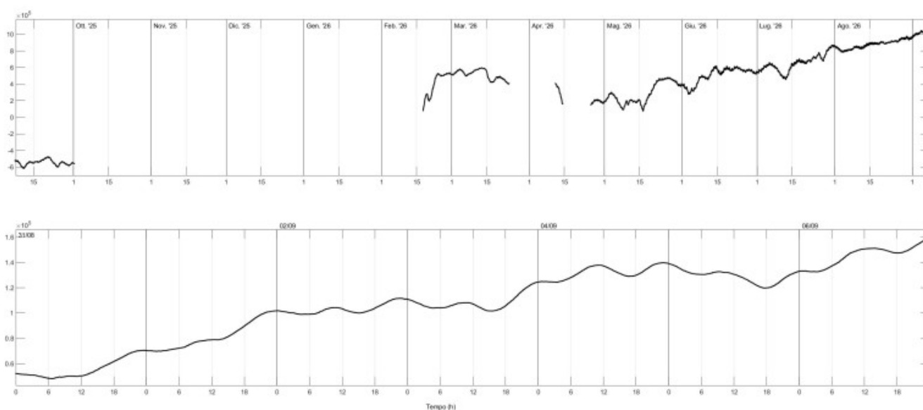
Fig. 4.3 Grafico relativo al dato dilatometrico registrato a SVO: in alto viene mostrato lo strain registrato nell'ultimo anno dal 08/09/2025; in basso quello registrato nell'ultima settimana.
