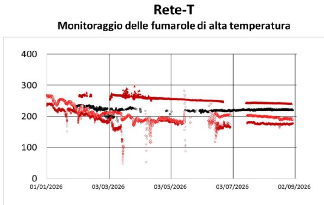
Fig. 3.1 Serie temporale dei valori di temperatura (°C) misurati in continuo nelle fumarole site sull'orlo del versante nord del cono La Fossa.
