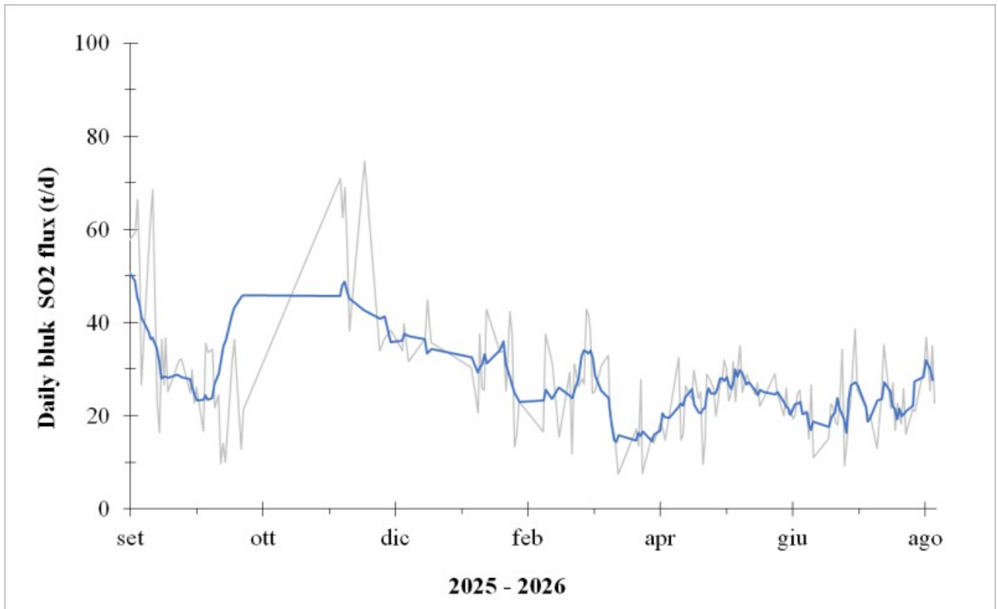
Fig. 5.1 Il flusso di SO 2 medio-giornaliero e medio-settimanale emesso dal campo fumarolico craterico di Vulcano nell'ultimo anno (rispettivamente, linea grigia e blu)
