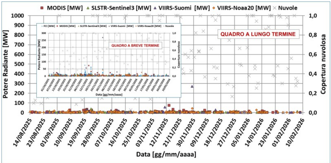
Fig. 7.1 Potere radiante calcolato da dati MODIS (quadrato rosso), SENTINEL-3 SLSTR (triangolo verde), VIIRS (triangolo viola e rombo giallo) e MTG-FCI (triangolo blu) dal 14 agosto 2025 al 10 febbraio 2026.
