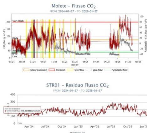
Fig. 6.5 Andamento del flusso medio giornaliero di CO 2 dal suolo registrato a Mofete (corretto per i parametri ambientali, linea rossa, grafico in alto) ed a Scari (grafico in basso) negli ultimi due anni.
