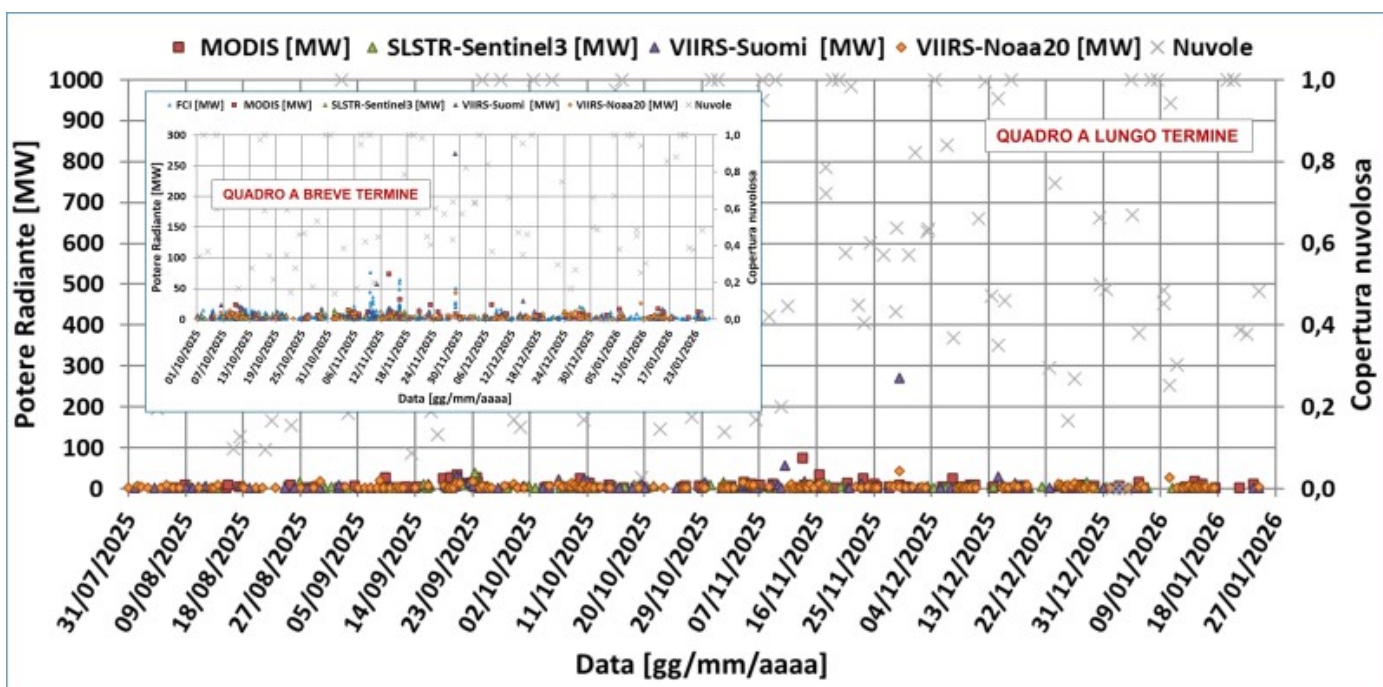
Fig. 7.1 Potere radiante calcolato da dati MODIS (quadrato rosso), SENTINEL-3 SLSTR (triangolo verde), VIIRS (triangolo viola e rombo giallo) e MTG-FCI (triangolo blu) dal 31 luglio 2025 al 27 gennaio 2026.
