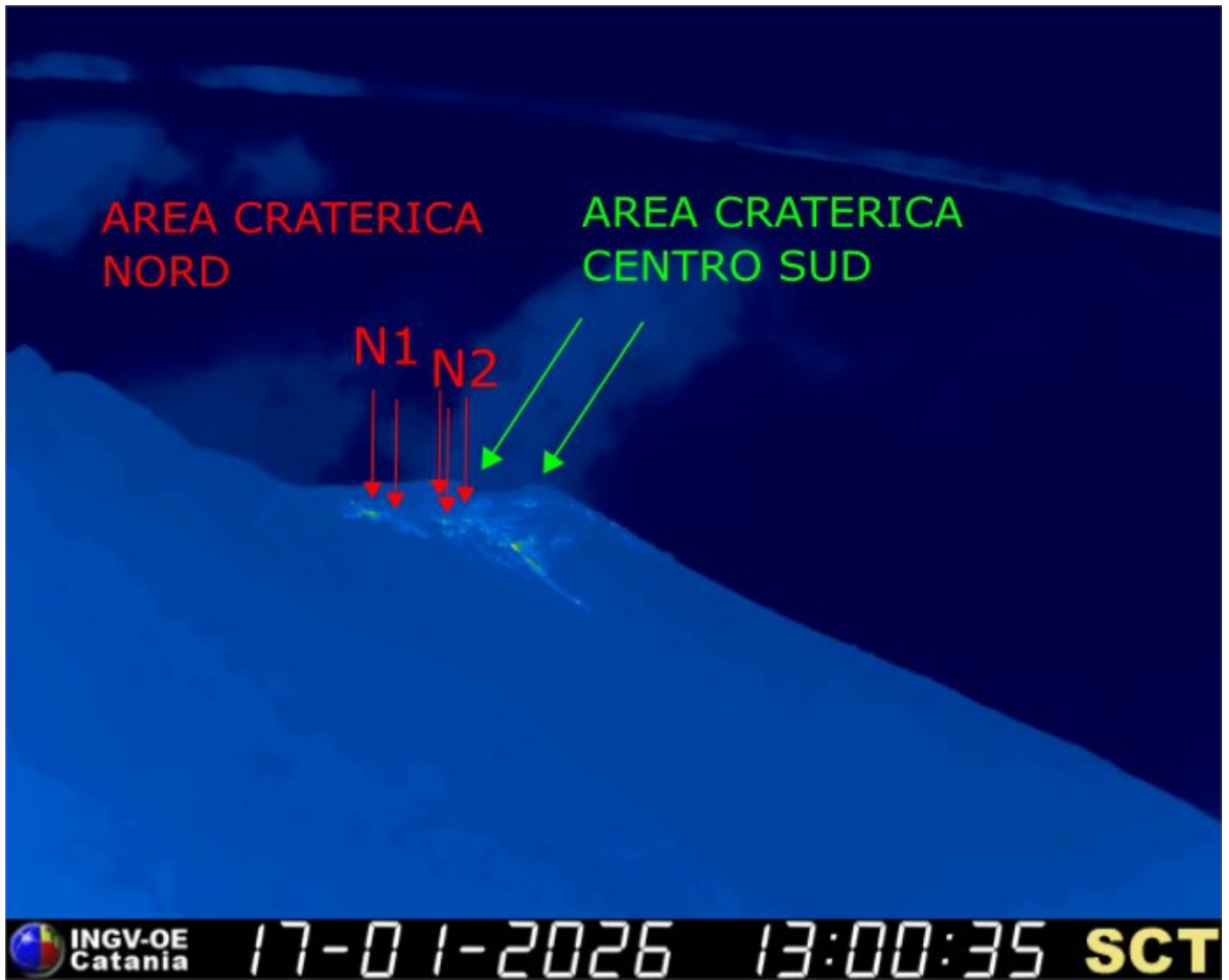
Fig. 3.1 La terrazza craterica vista dalla telecamera termica posta a quota 190 con la delimitazione delle aree crateriche Area Centro-Sud e Area Nord. Le frecce indicano le bocche attive.
