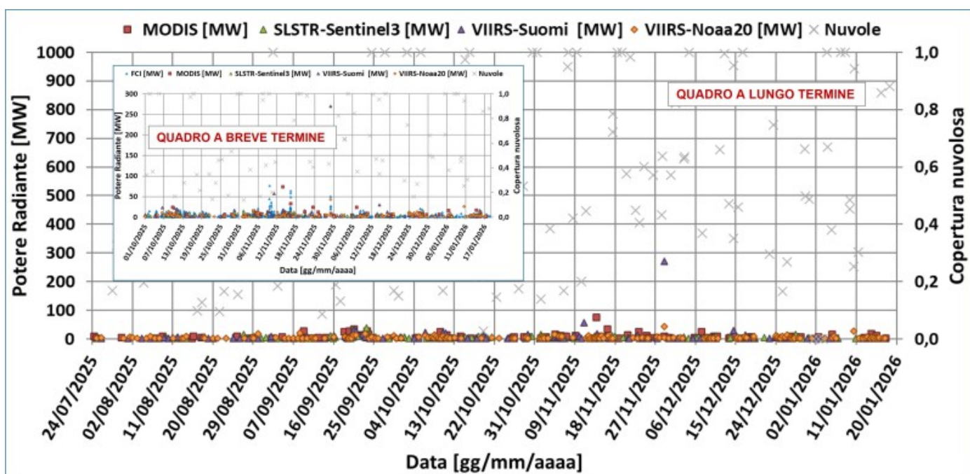
Fig. 7.1 Potere radiante calcolato da dati MODIS (quadrato rosso), SENTINEL-3 SLSTR (triangolo verde), VIIRS (triangolo viola e rombo giallo) e MTG-FCI (triangolo blu) dal 24 luglio 2025 al 20 gennaio 2026.
