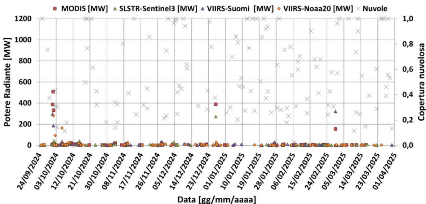
Fig. 7.1 Potere radiante calcolato da dati MODIS (quadrato rosso), SENTINEL-3 SLSTR (triangolo verde) e VIIRS (triangolo viola e rombo giallo) dal 24 settembre 2024 al 1° aprile 2025.
