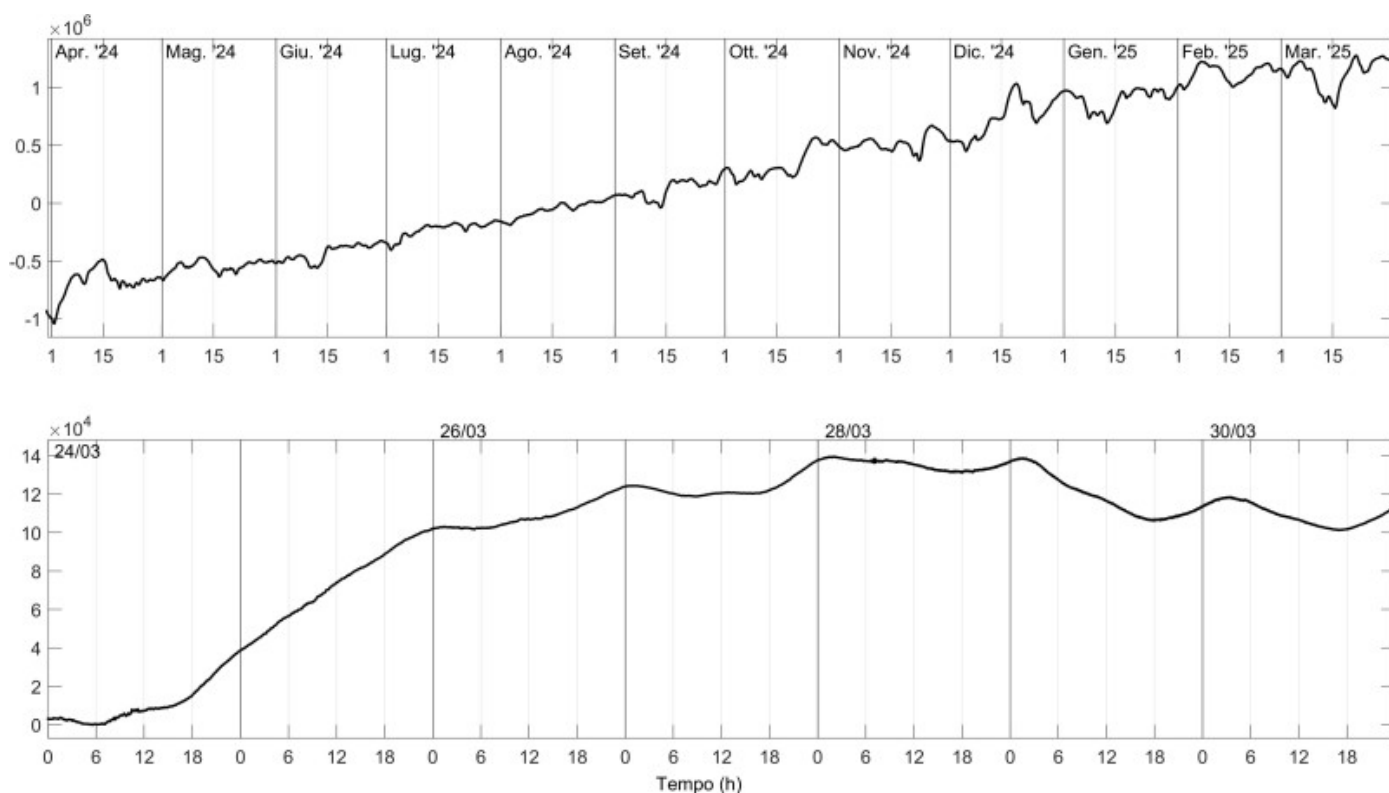
Fig. 4.3 Grafico relativo al dato dilatometrico registrato a SVO: in alto viene mostrato lo strain registrato nell'ultimo anno dal 31/03/2024; in basso quello registrato nell'ultima settimana.
