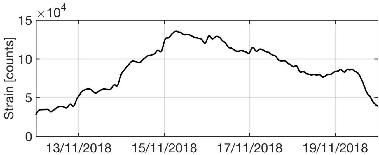
Fig. 4.4 - Grafico relativo ai dati dilatometrici registrati a SVO: in nero viene mostrato il dato processato, ripulito dalle maree.
