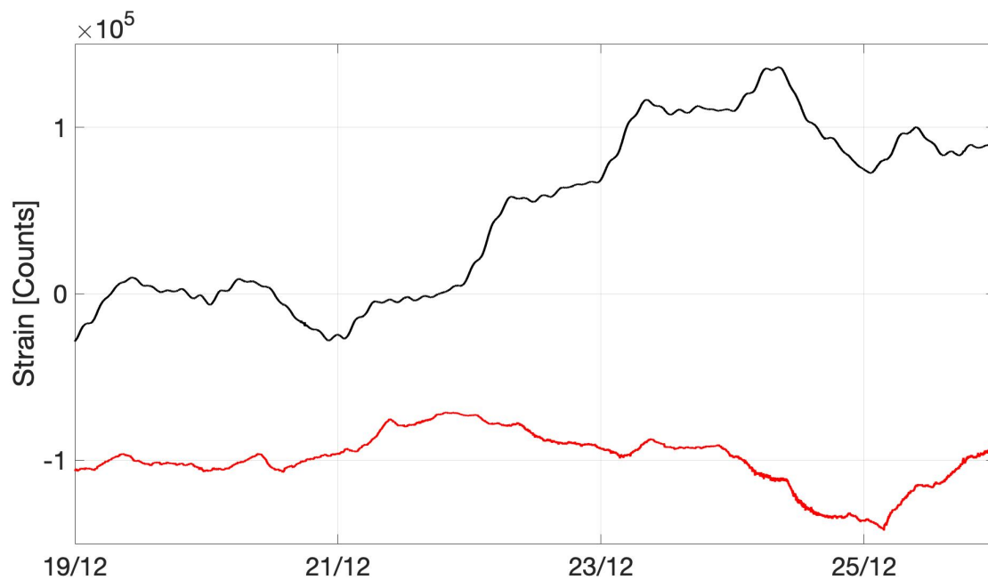
Fig. 4.4 - Grafico relativo ai dati dilatometrici registrati a SVO: in nero viene mostrato il dato ripulito dalle maree, mentre in rosso l'andamento della pressione atmosferica.
